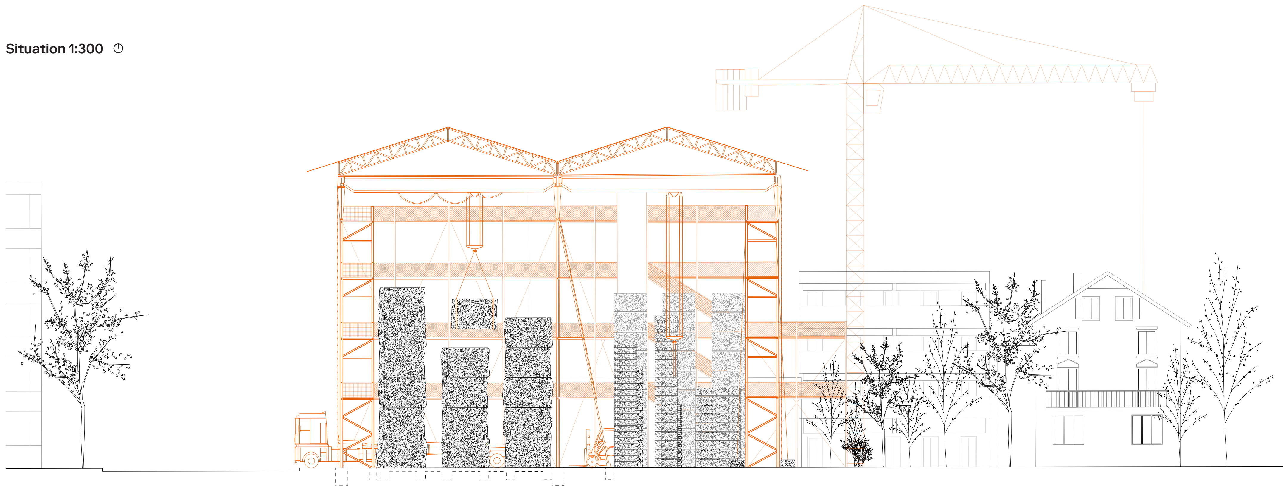
Schnitt 1:150
