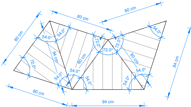
Grundriss 1 : 20
