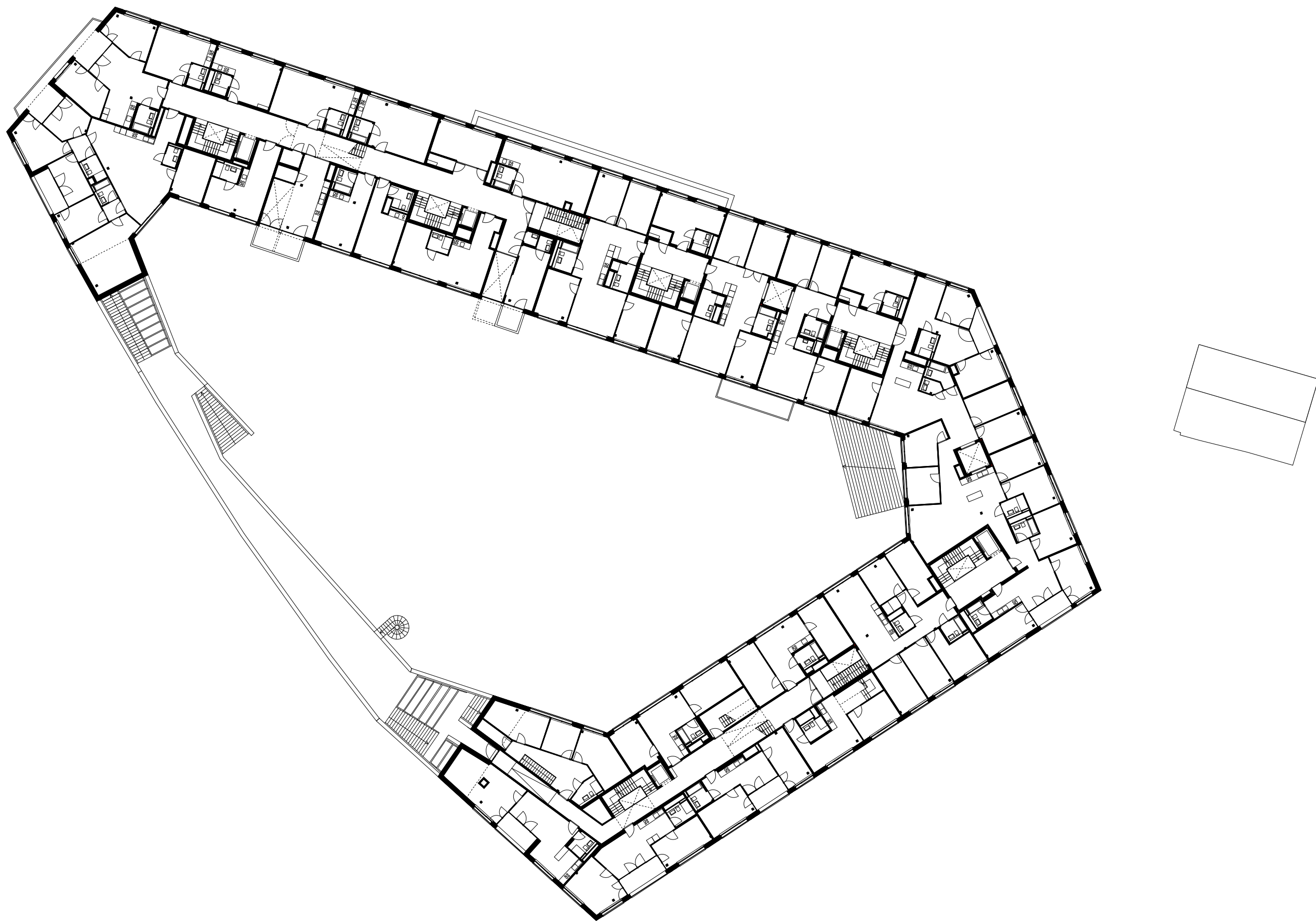
GRUNDRISS 4. OBERGESCHOSS 1:400
