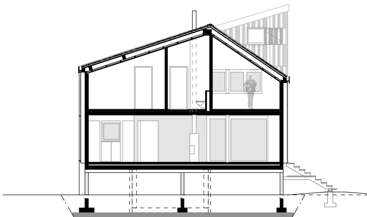
1 2.5 5 COUPE TRANSVERSALE - SEJOUR
