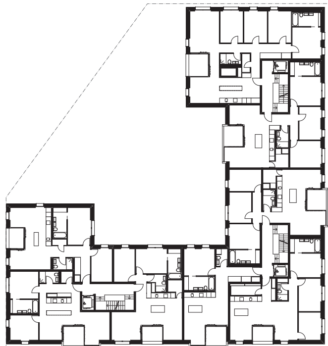
HAUS A
