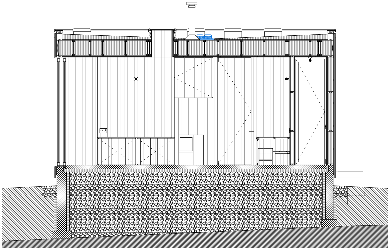
SCHNITT Z - Z
