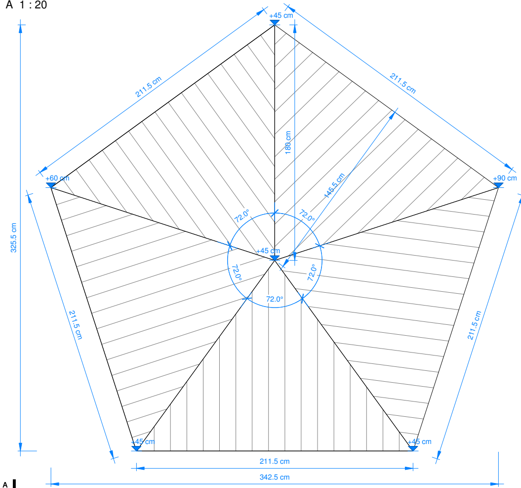
Grundriss 1 : 20
