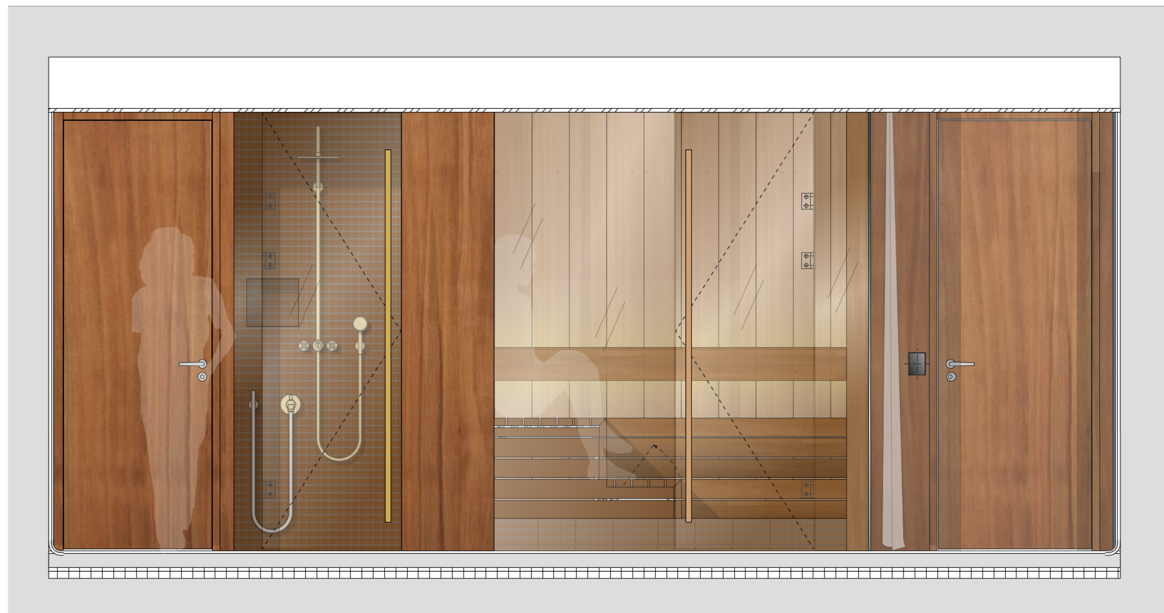
Ansicht A-A | Mst. 1:20
