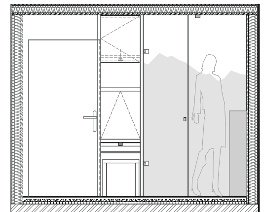
queransicht
