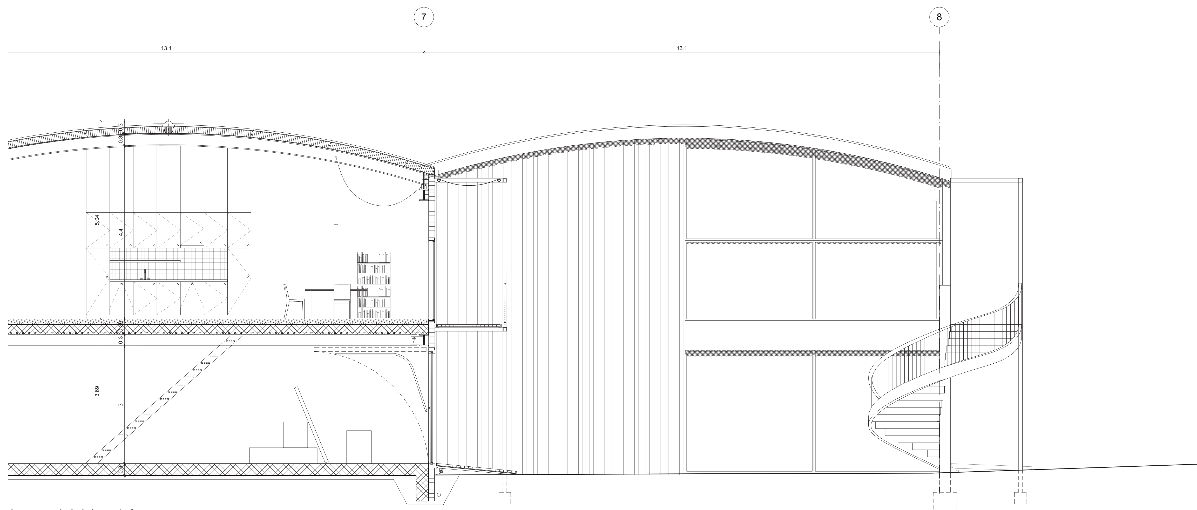
Coupe transversale - Duplex logement/atelier Warehouse, 1:50
