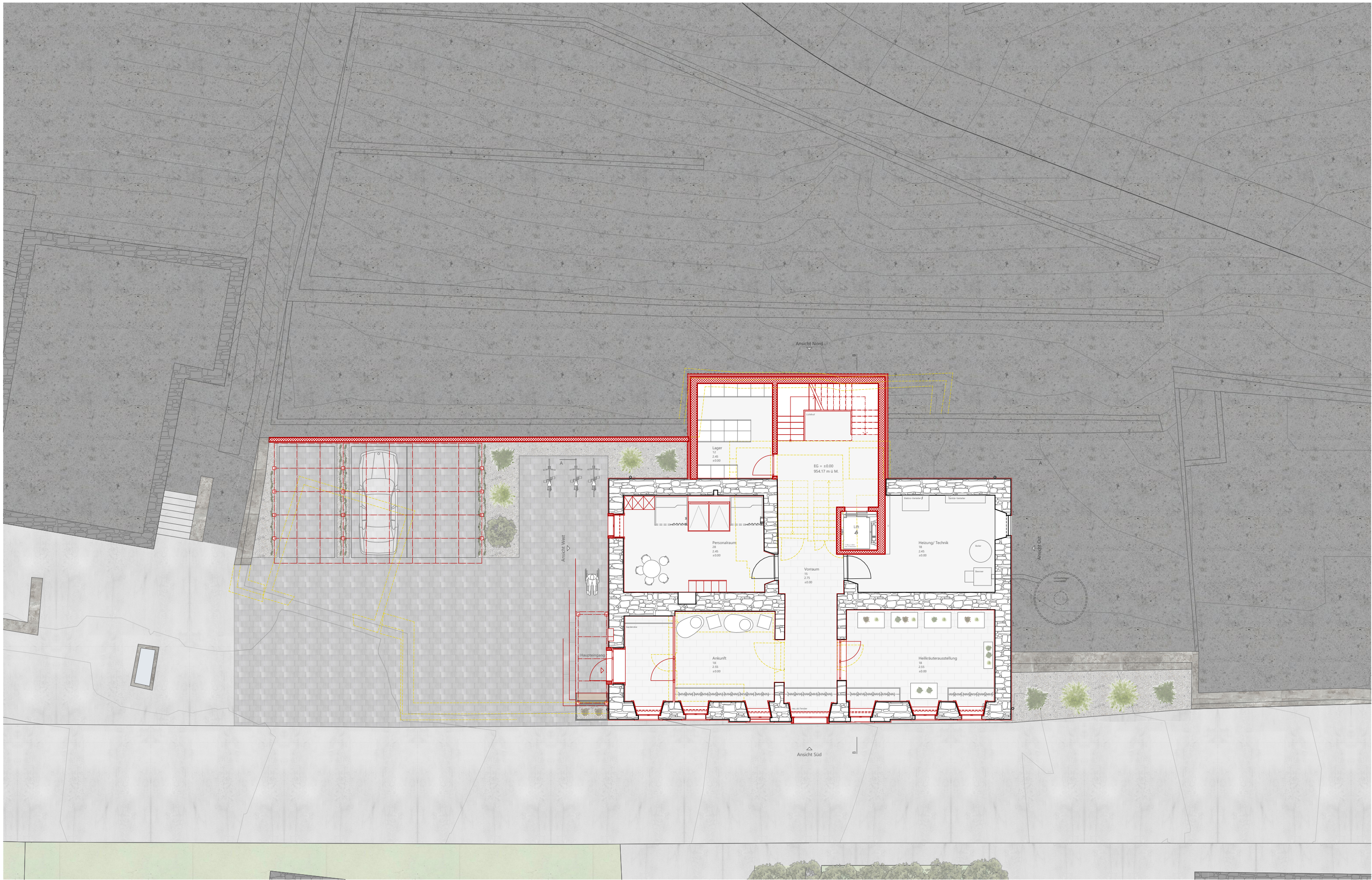
Erdgeschoss | 1:150
