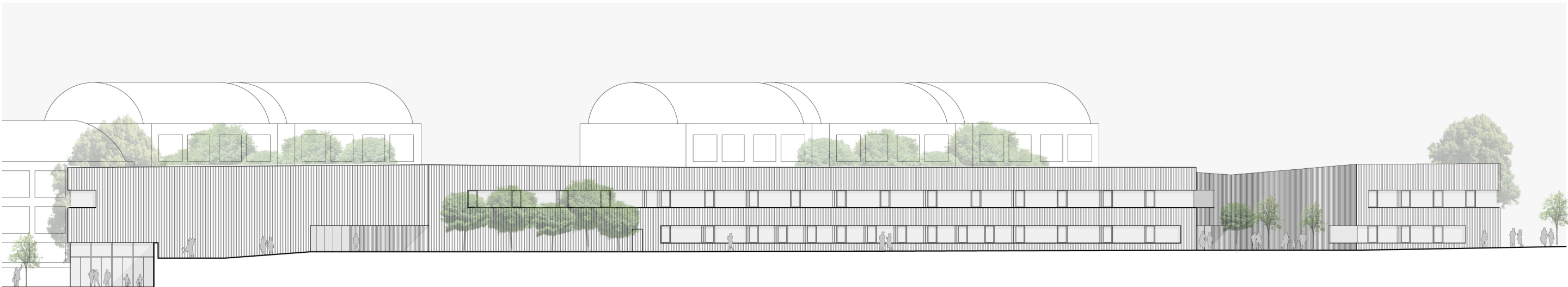
ELEVATION SUD EXT.
