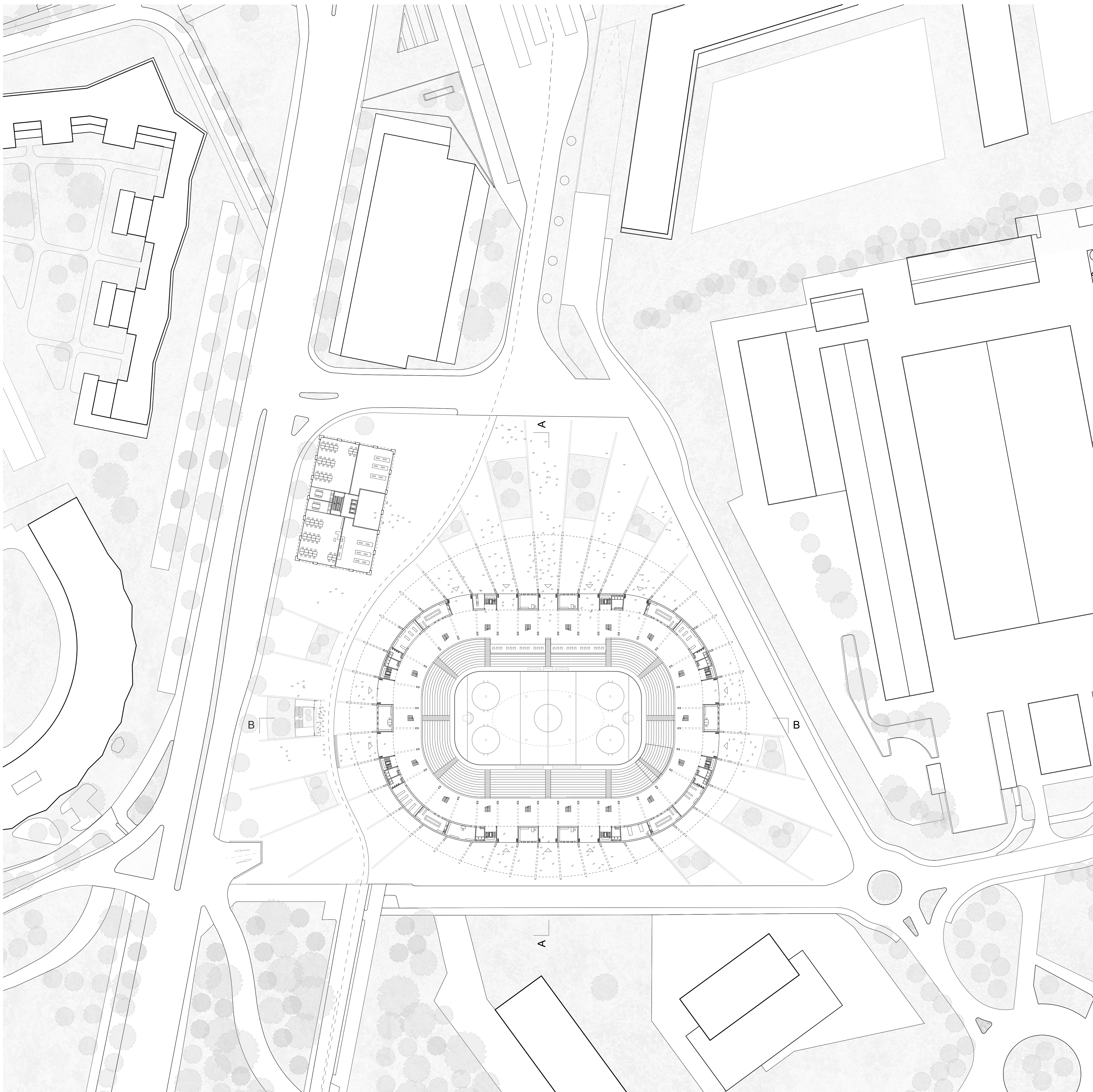
Plan du niveau 0
