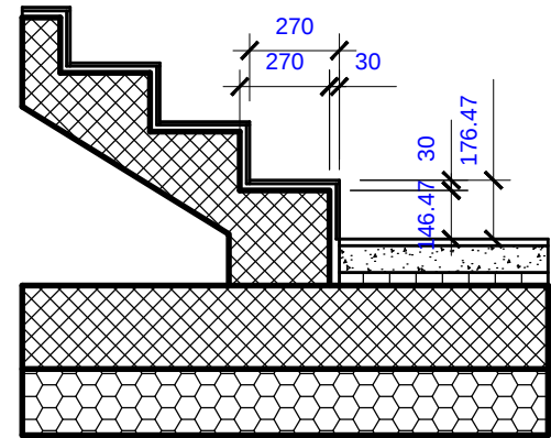
Detail D5
