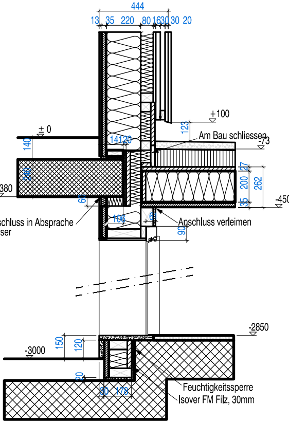
Detail D2
