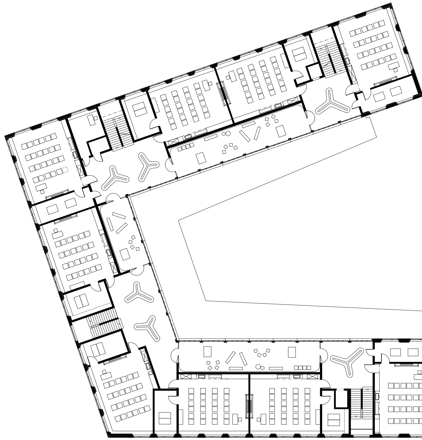
1. Obergeschoss
