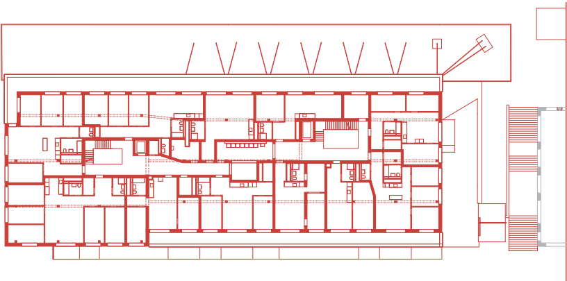
3. Obergeschoss | 3 ème étage
