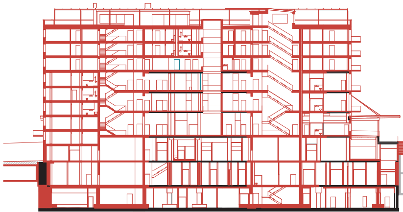
Schnitt A | Coupe A
