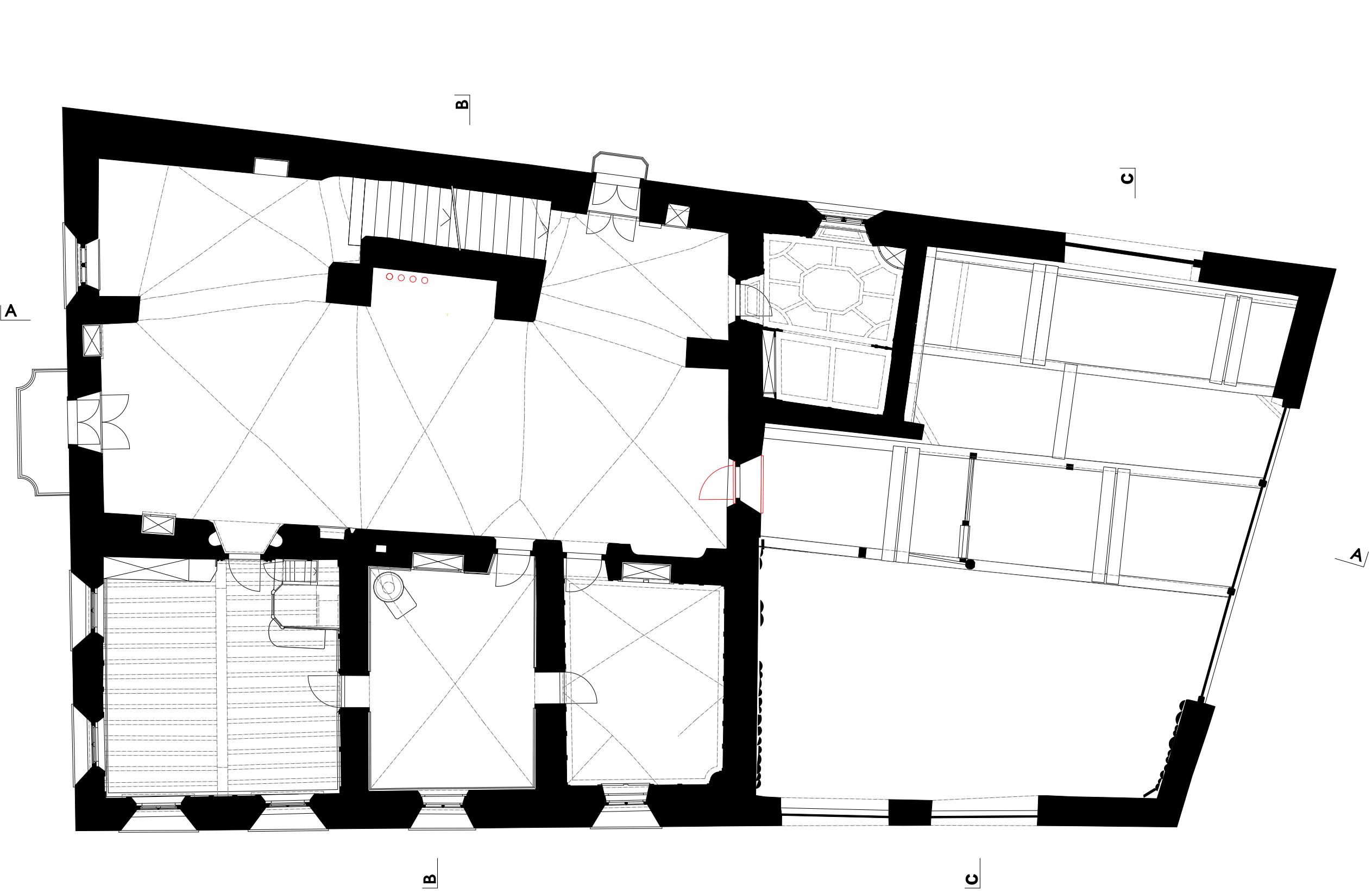
I. Obergeschoss
