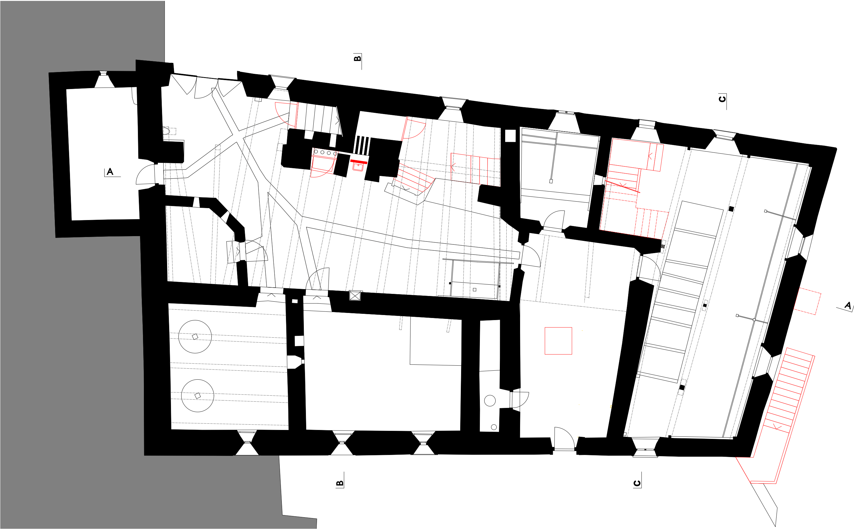
I. Untergeschoss
