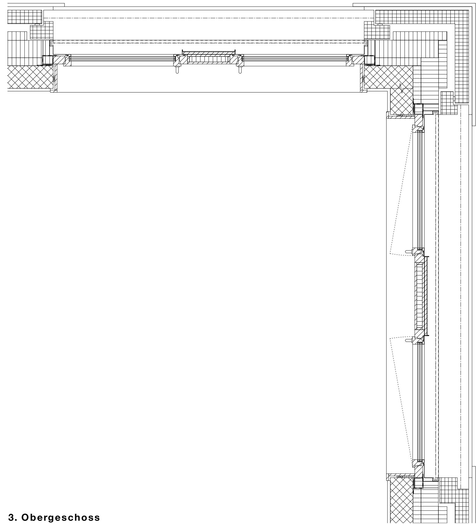
3. Obergeschoss
