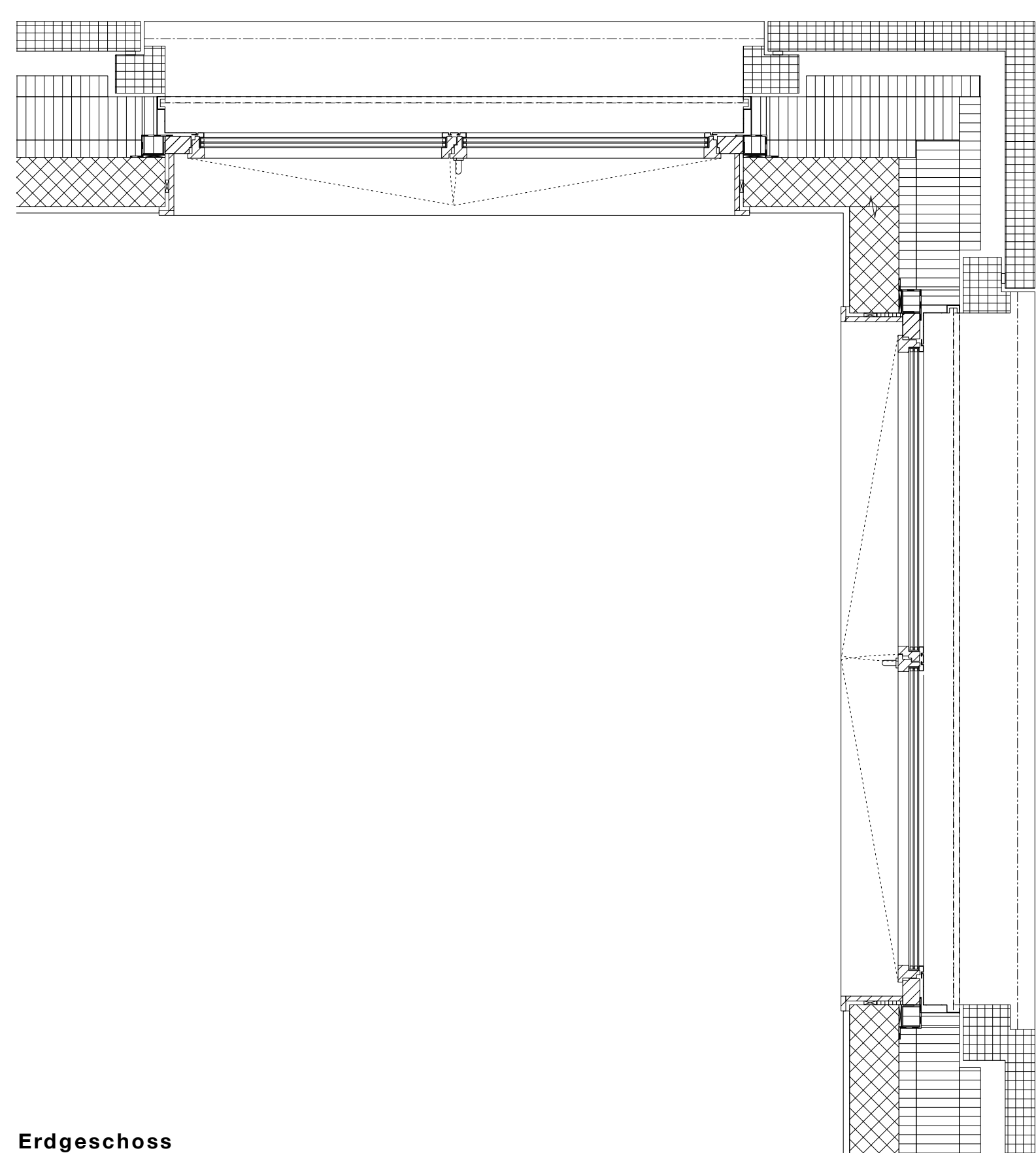
Erdgeschoss
