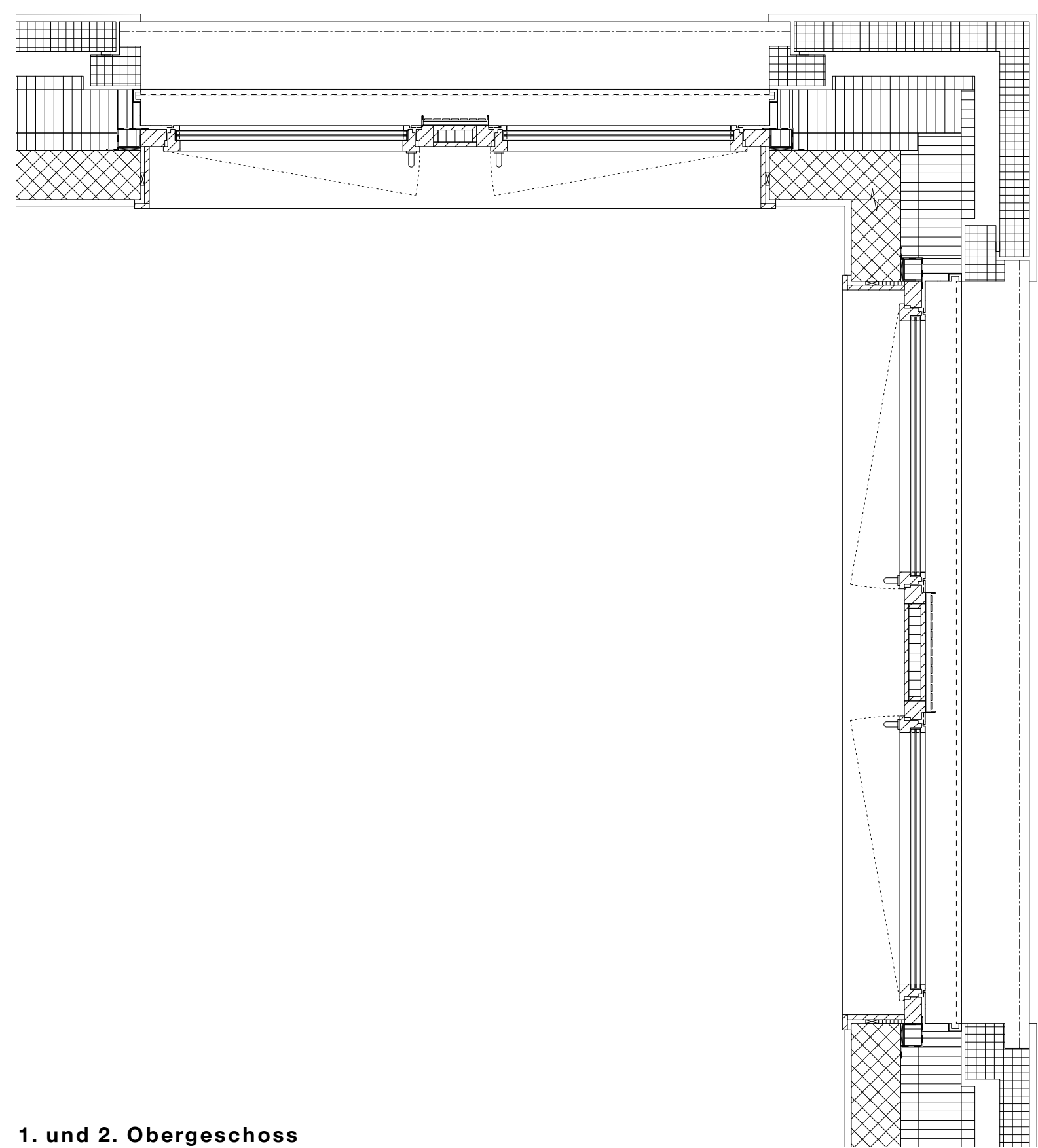
1. und 2. Obergeschoss
