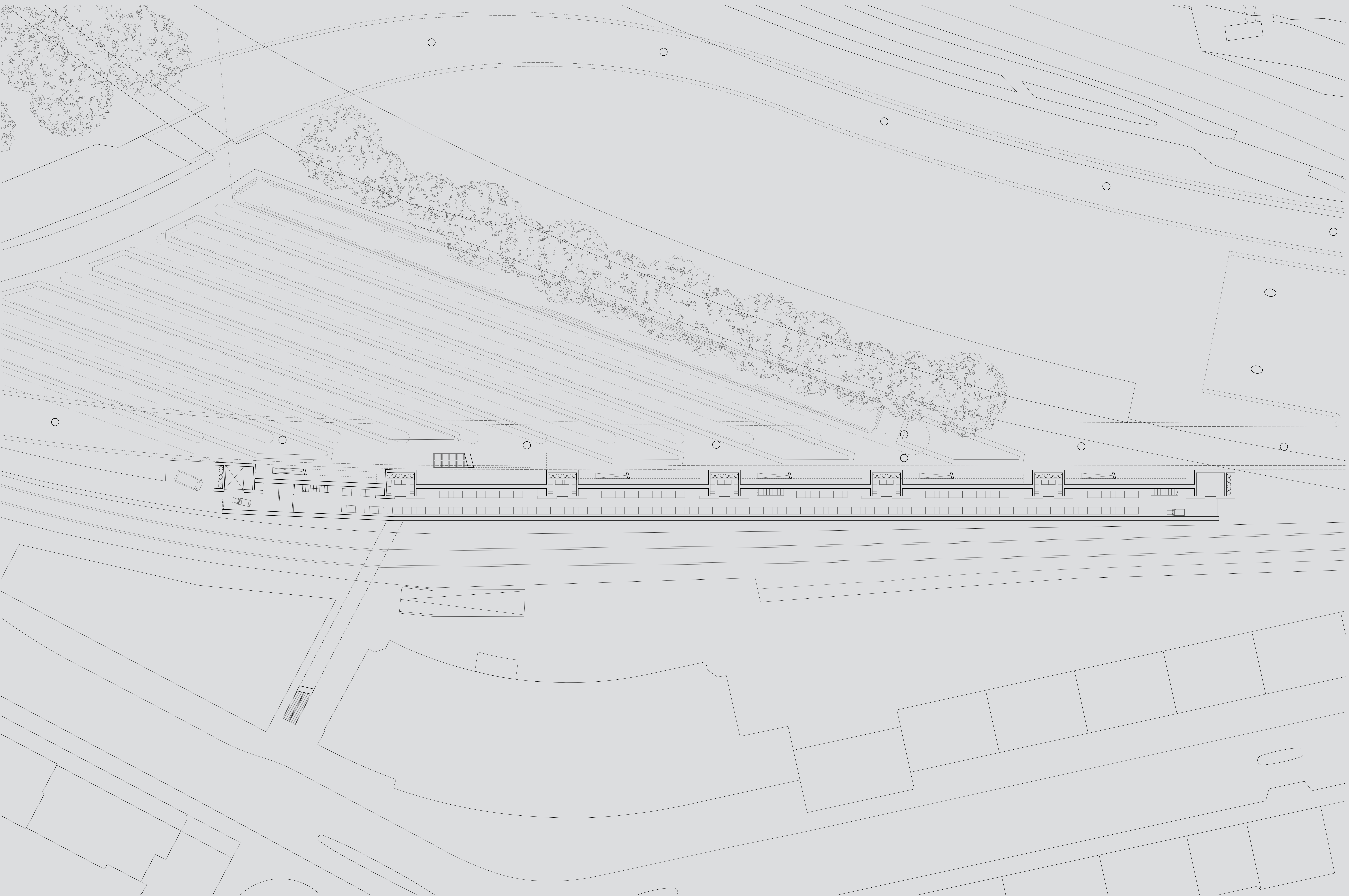
Erdgeschoss Rechenzentrum 1 : 200
