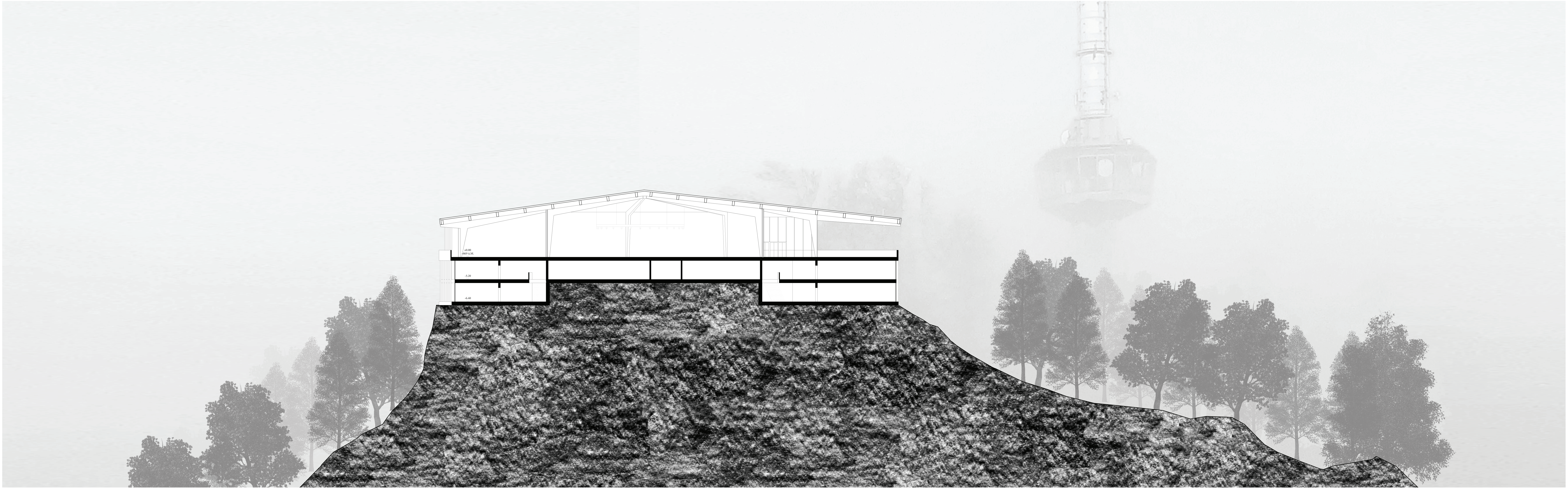
Schnitt Quer 1:200
