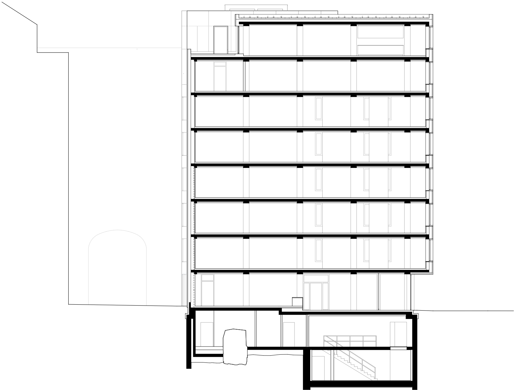
Schnitt C-C, 1:200 0 1 2 5 10
