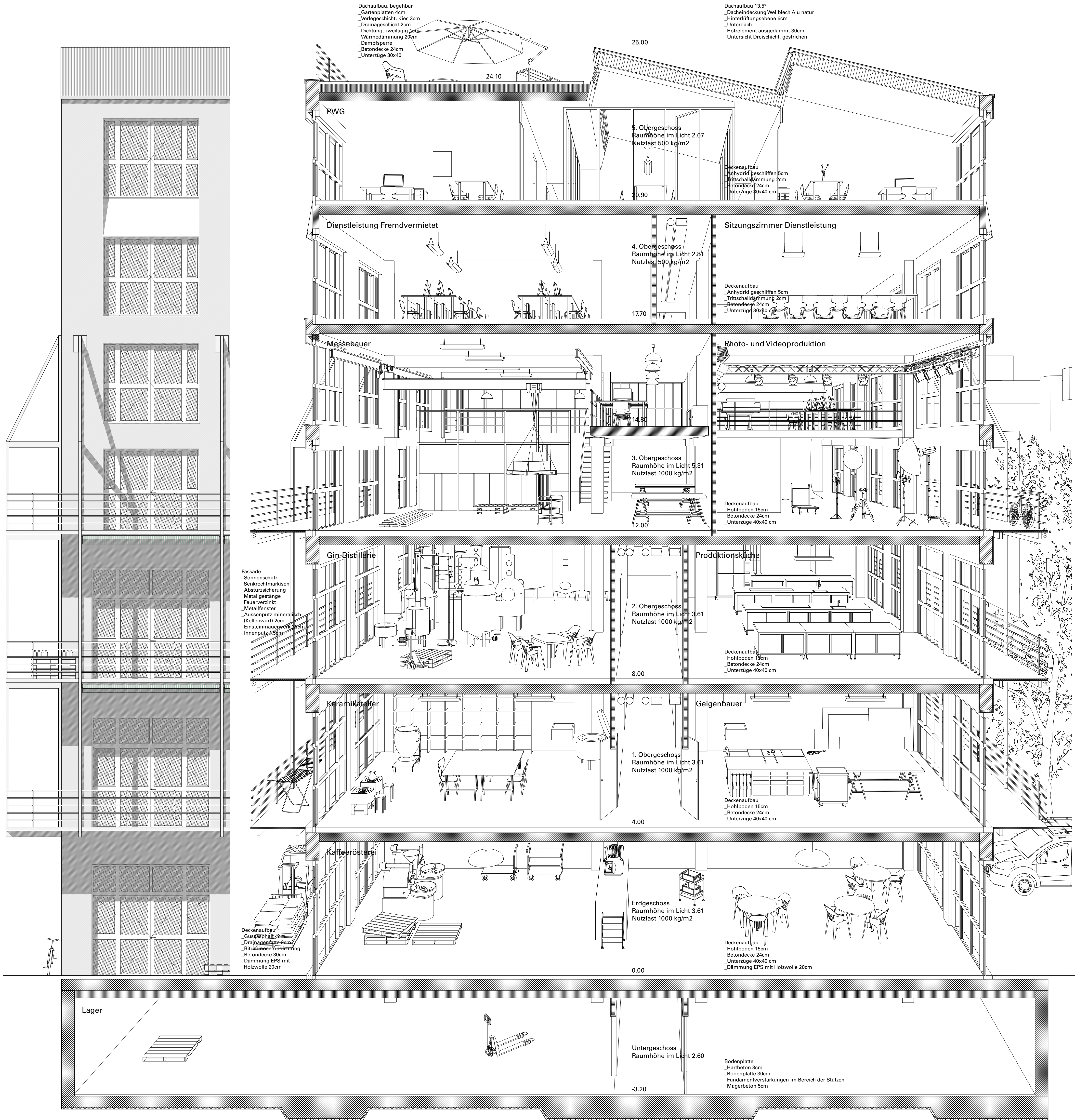
Konstruktionsschnitt, Fassade 1:50
