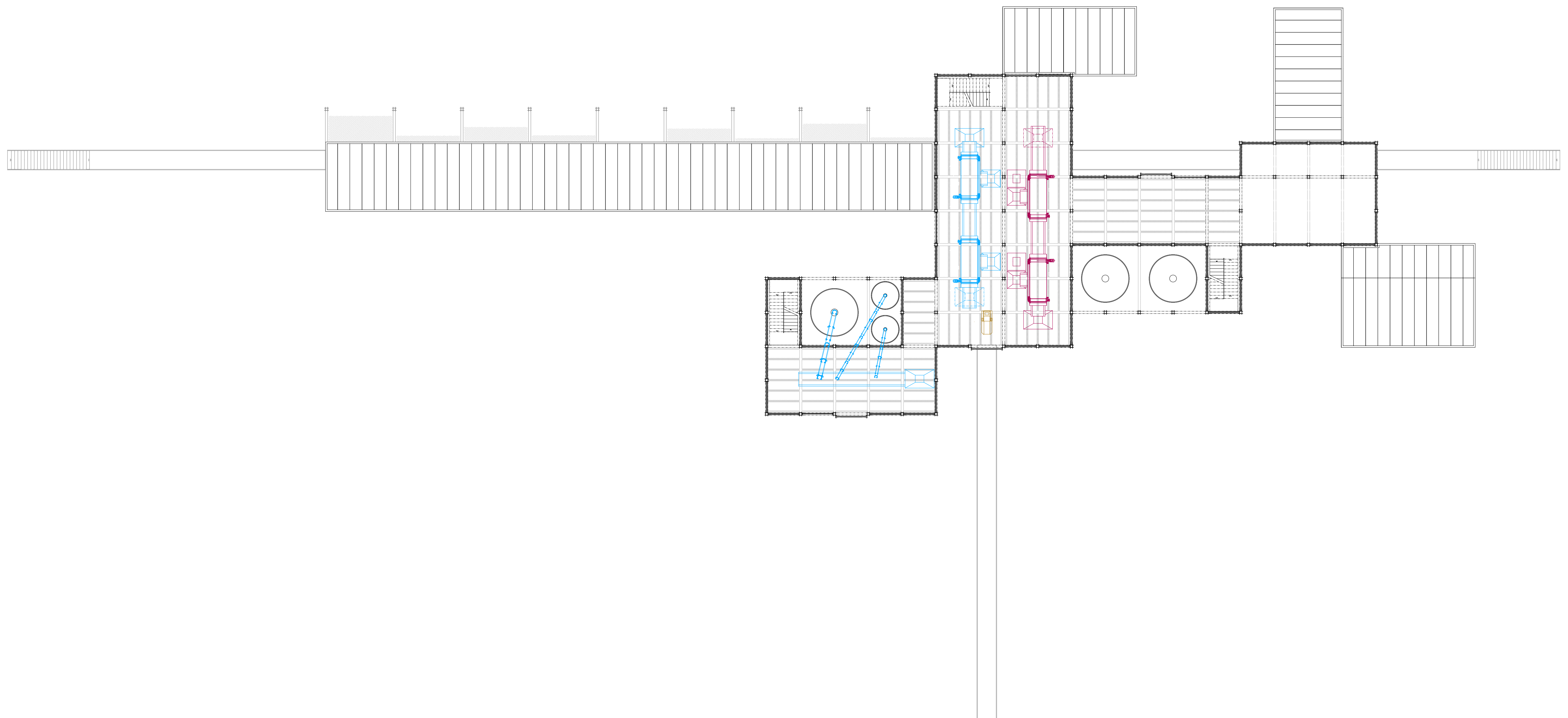
Grundriss 3.Obergeschoss 1:200
