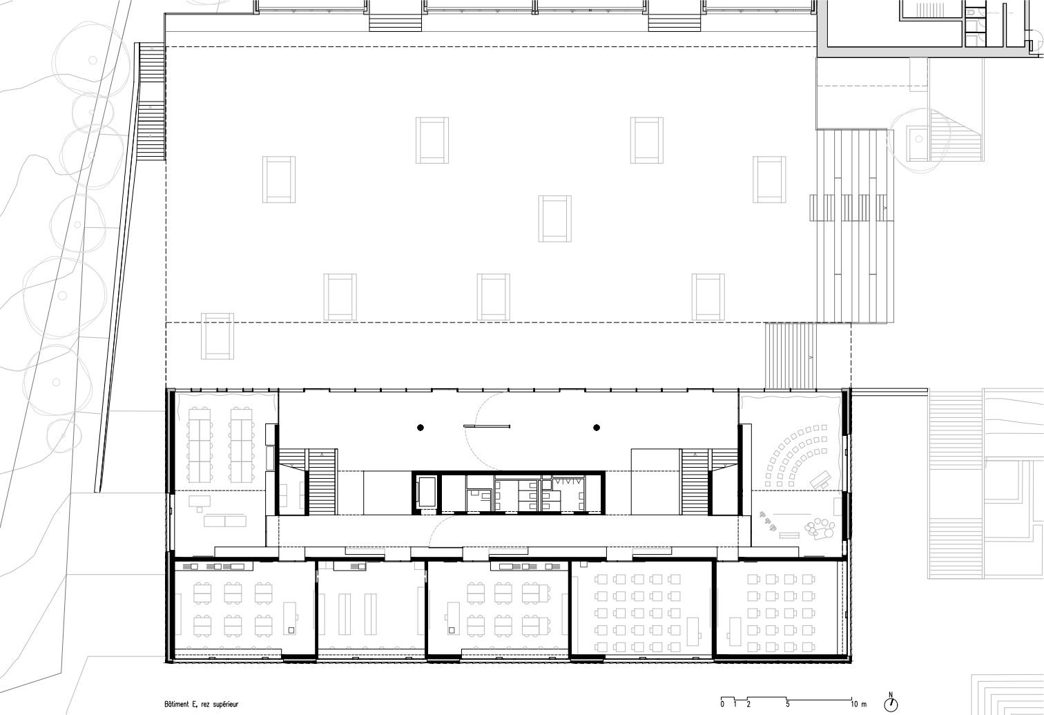
Bâtiment E, rez supérieur
