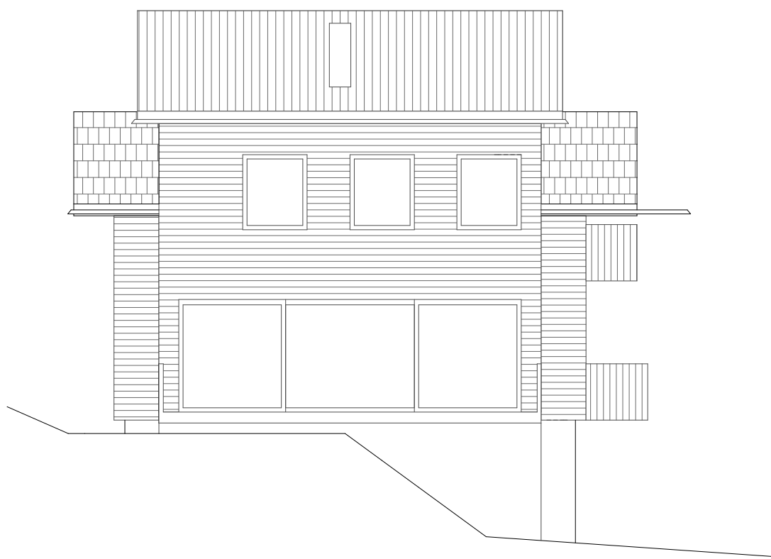
façade latérale
