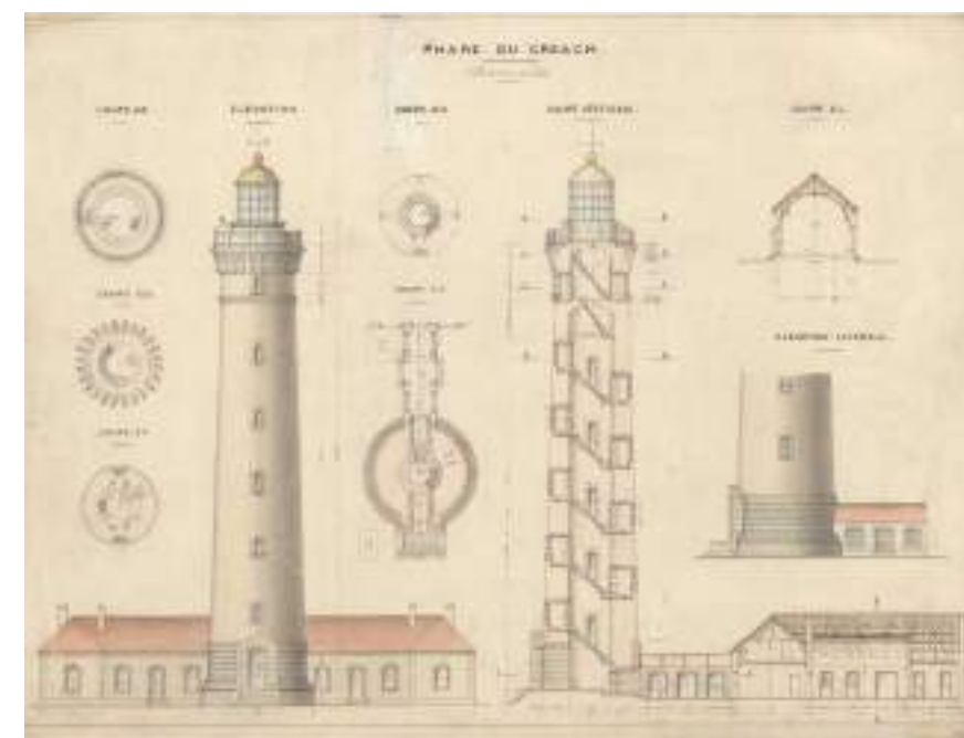
Phare du Crac'h sur l'île d'Ouessant en France . 1863 . h du feu: 70m
