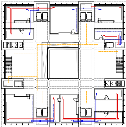
Gebäudetechnik Konzept
