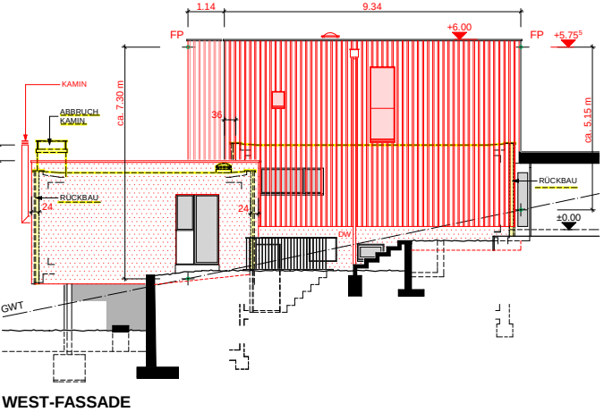
WEST-FASSADE
