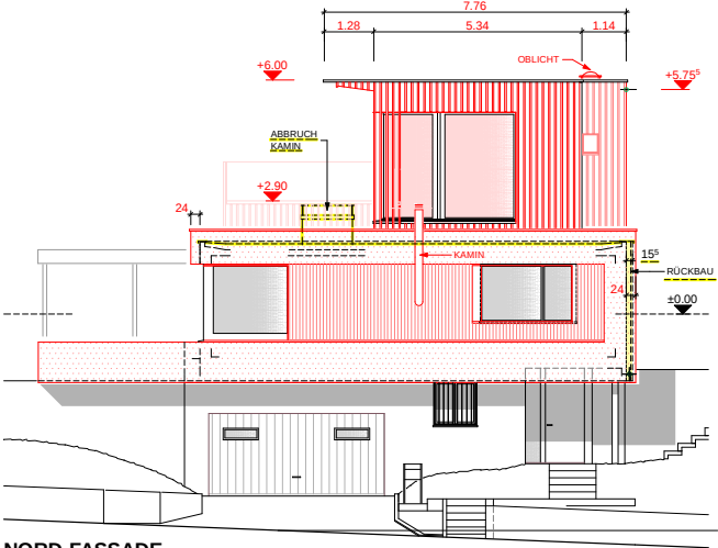
NORD-FASSADE
