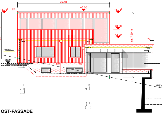
OST-FASSADE
