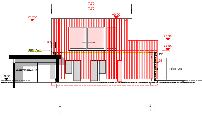
WEST-FASSADE
