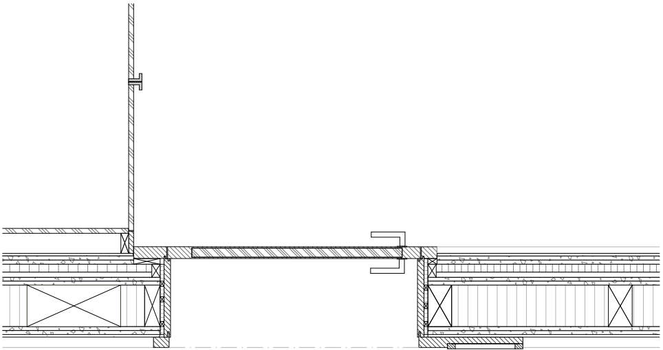
Grundriss
