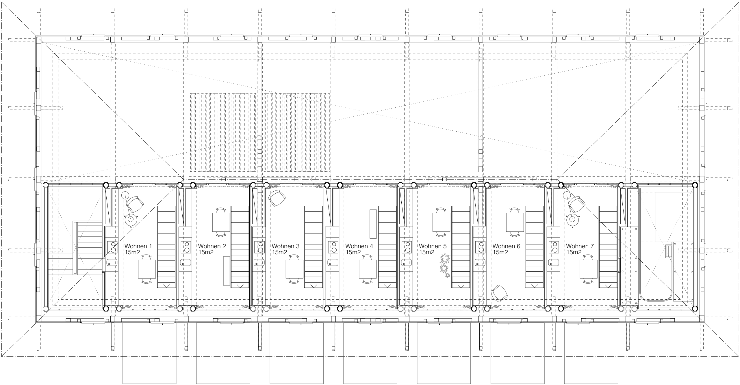
Dachgeschoss Niveau 2 1_100
