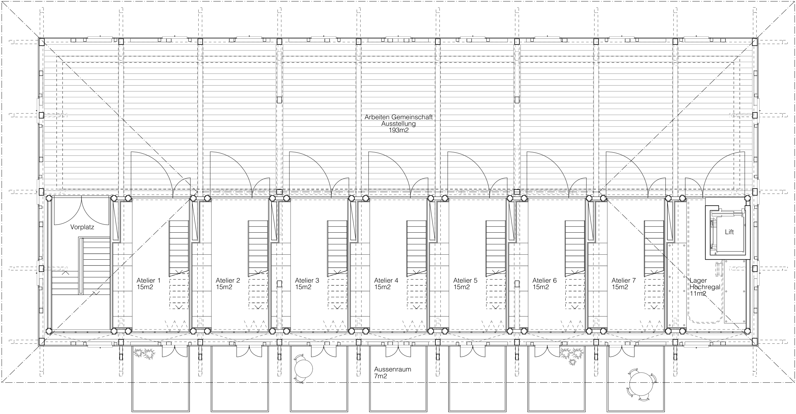
Dachgeschoss Niveau 1 1_100
