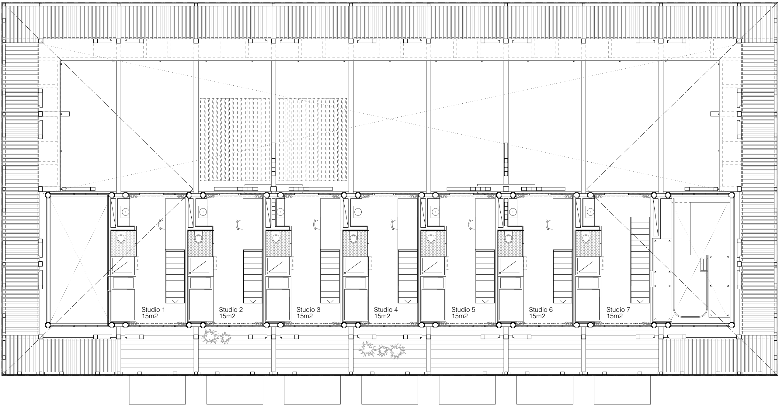
Dachgeschoss Niveau 3 1_100
