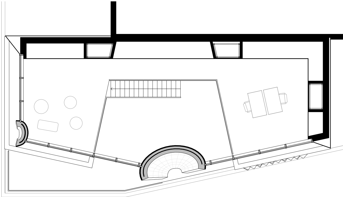
Grundriss Galerie M 1:100
