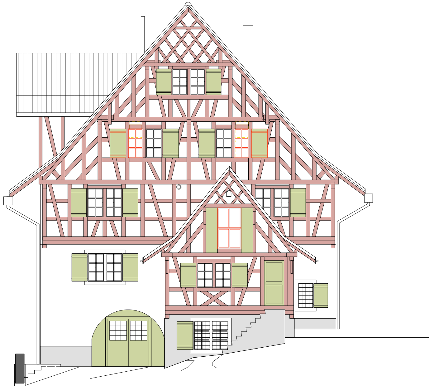
Ost-Fassade 1:100
