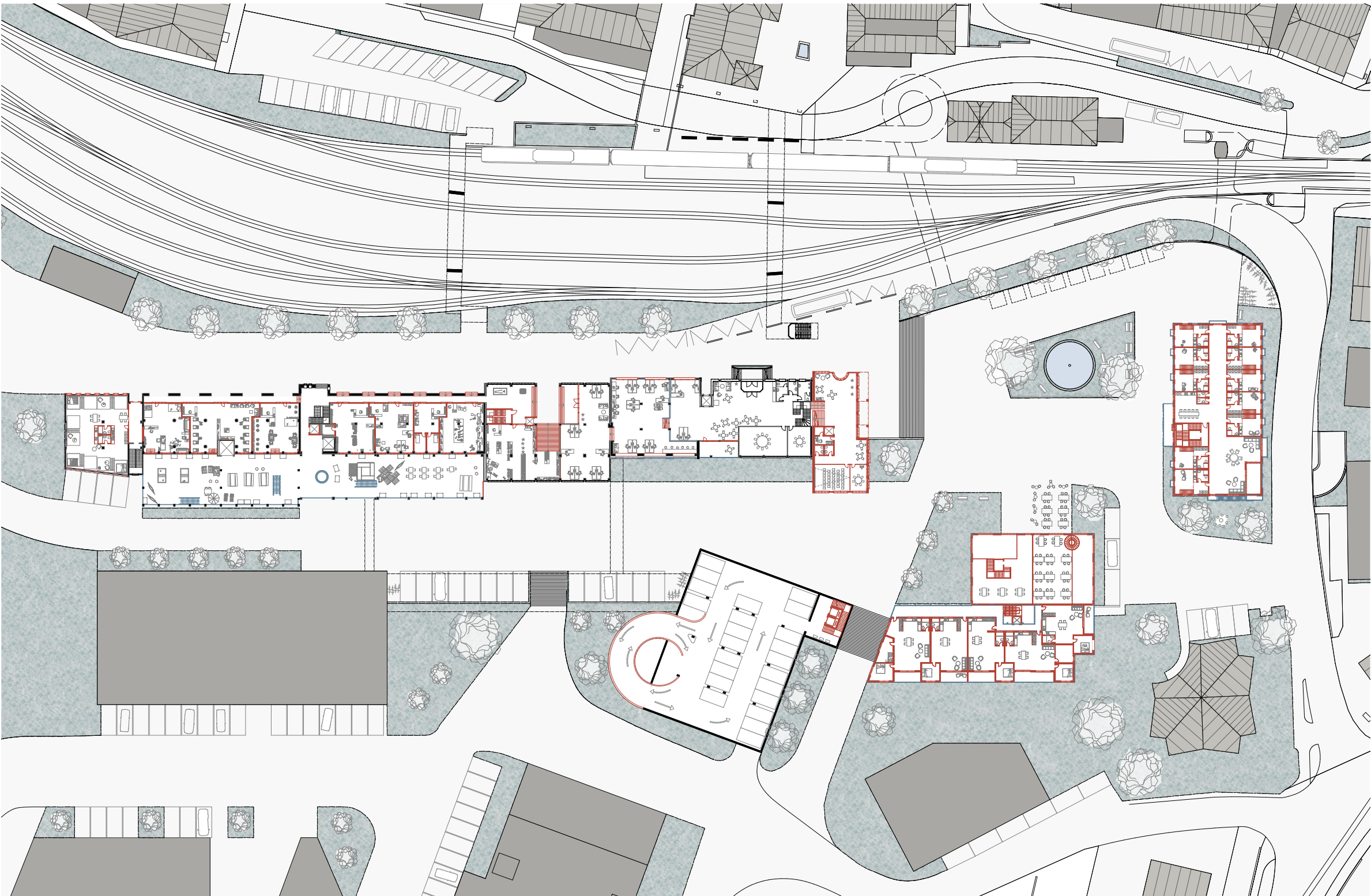
Grundriss, Niveau 0 Gleise
