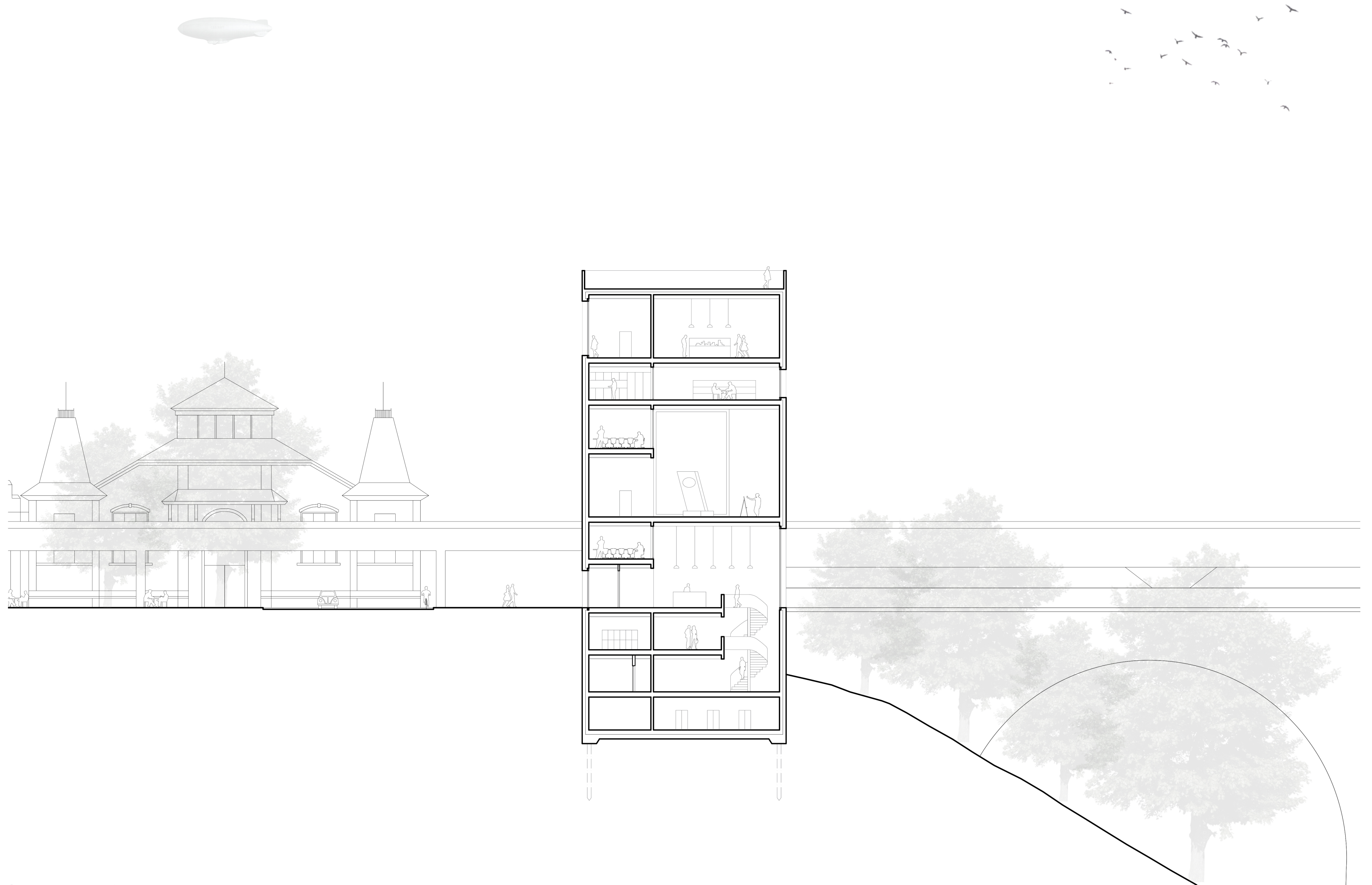
Coupe transversale 1/200
