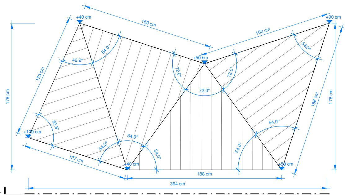
Grundriss 1 : 20
