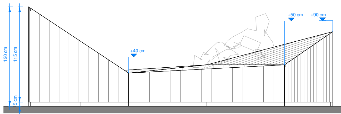
A 1 : 20
