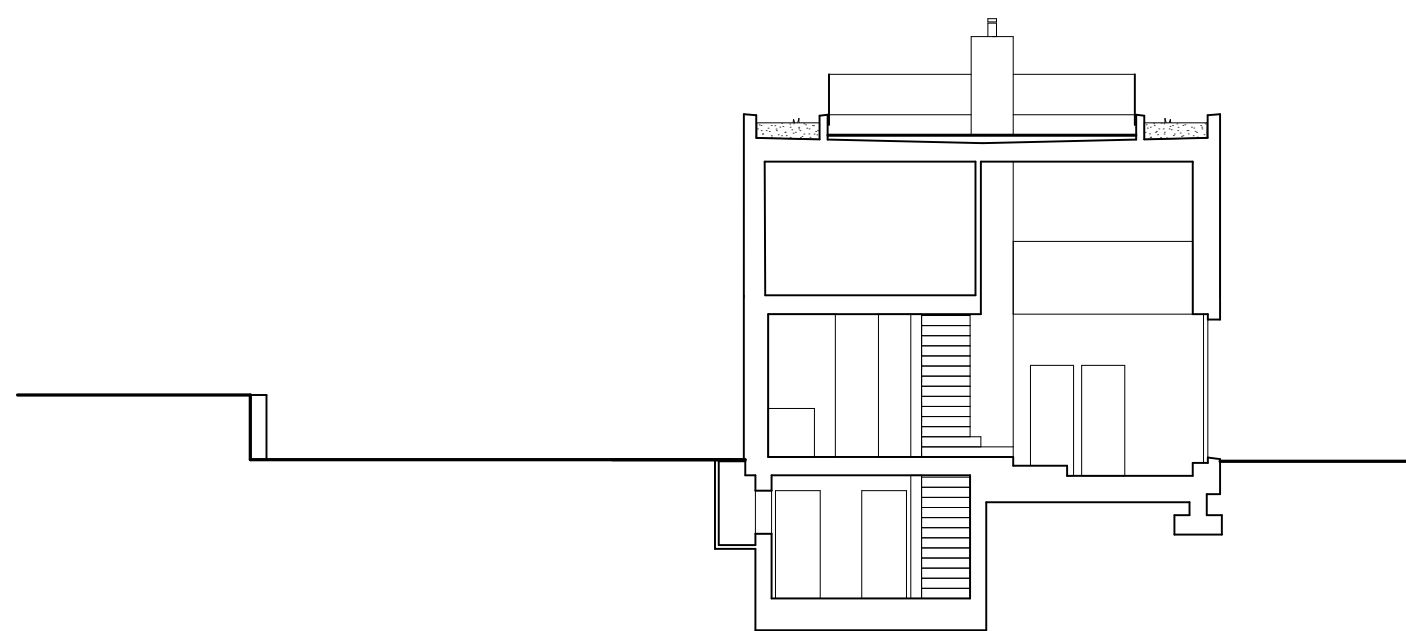
Coupe transversale
