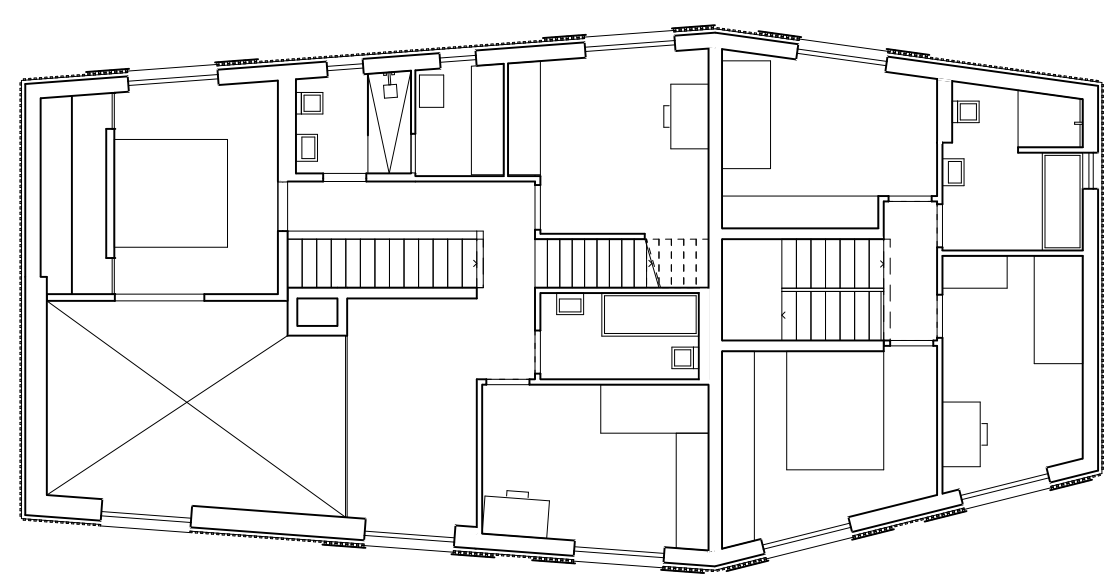
Etage
