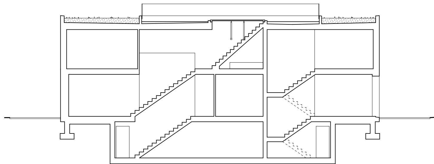
Coupe longitudinale
