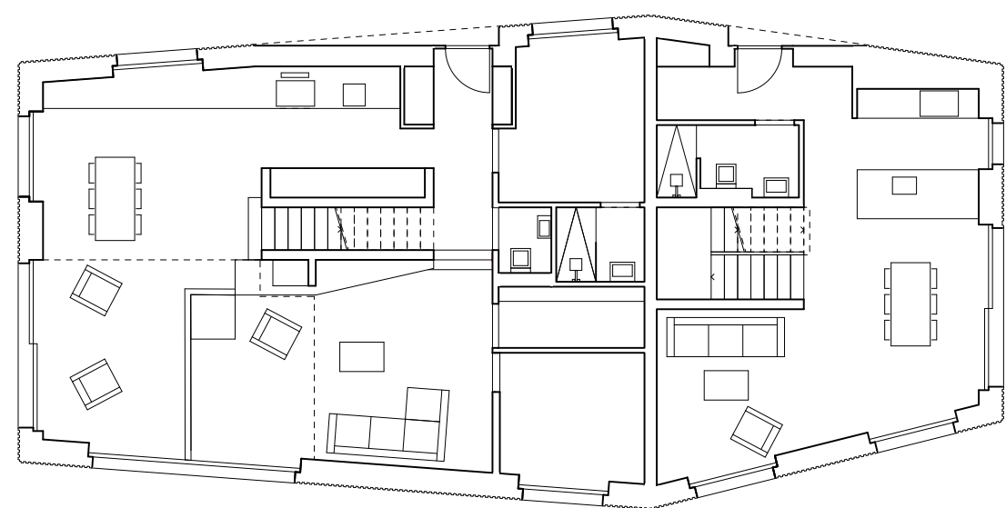
Rez-de-chaussée
