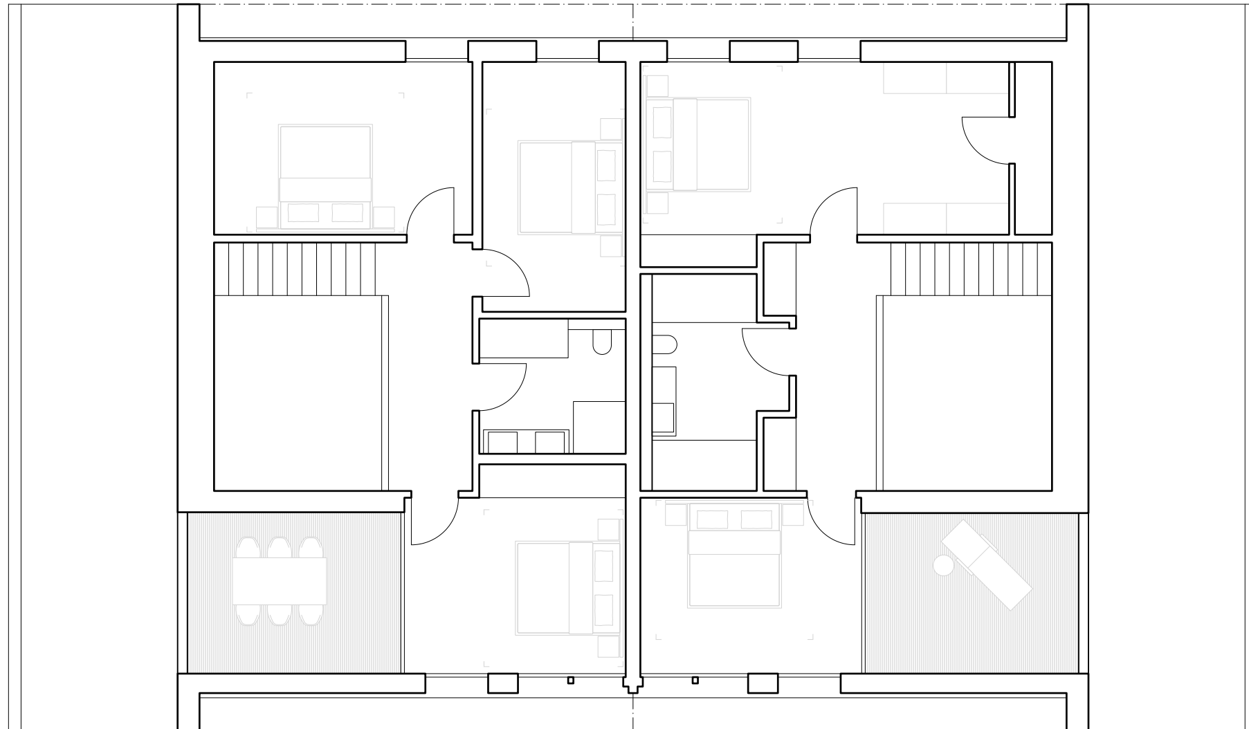
Grundriss Dachgeschoss 1:100
