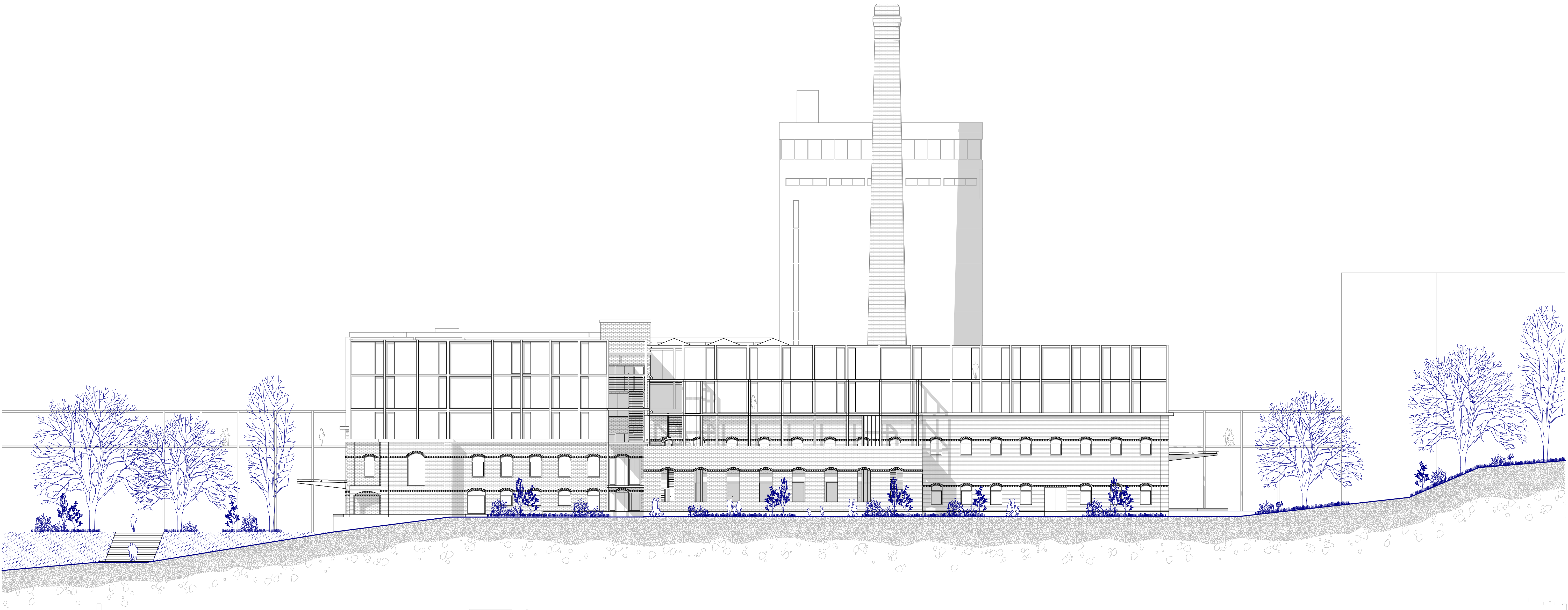
Façade Nord | échelle 1: 200
