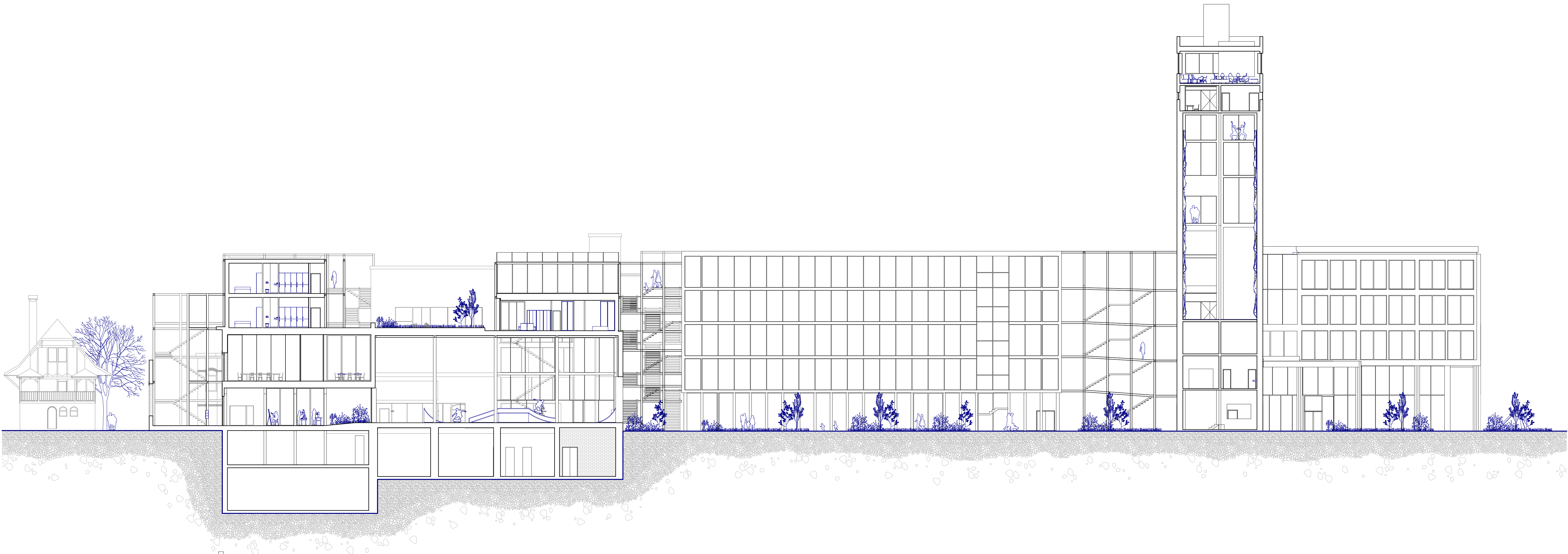
Façade Ouest | échelle 1: 200
