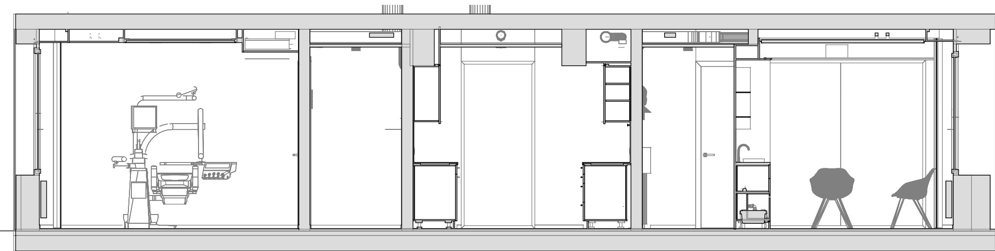
Schnitt C
