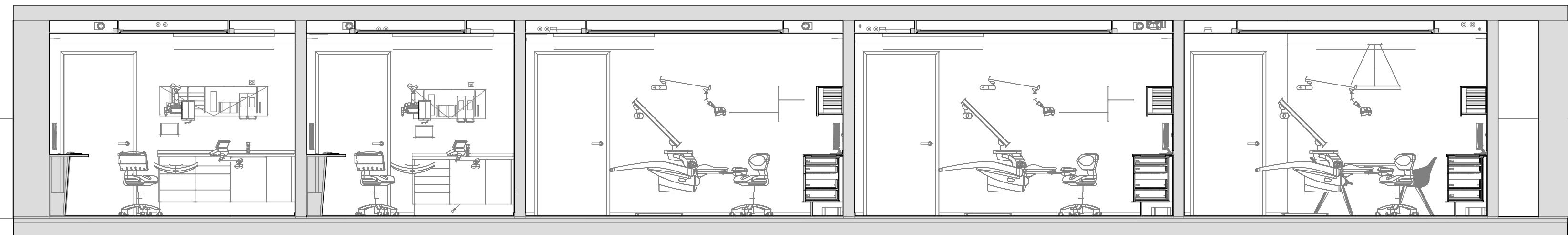
Schnitt D
