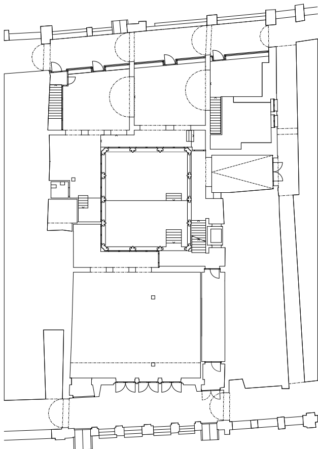
Erdgeschoss 1:400
