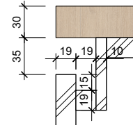
Poignée 2
