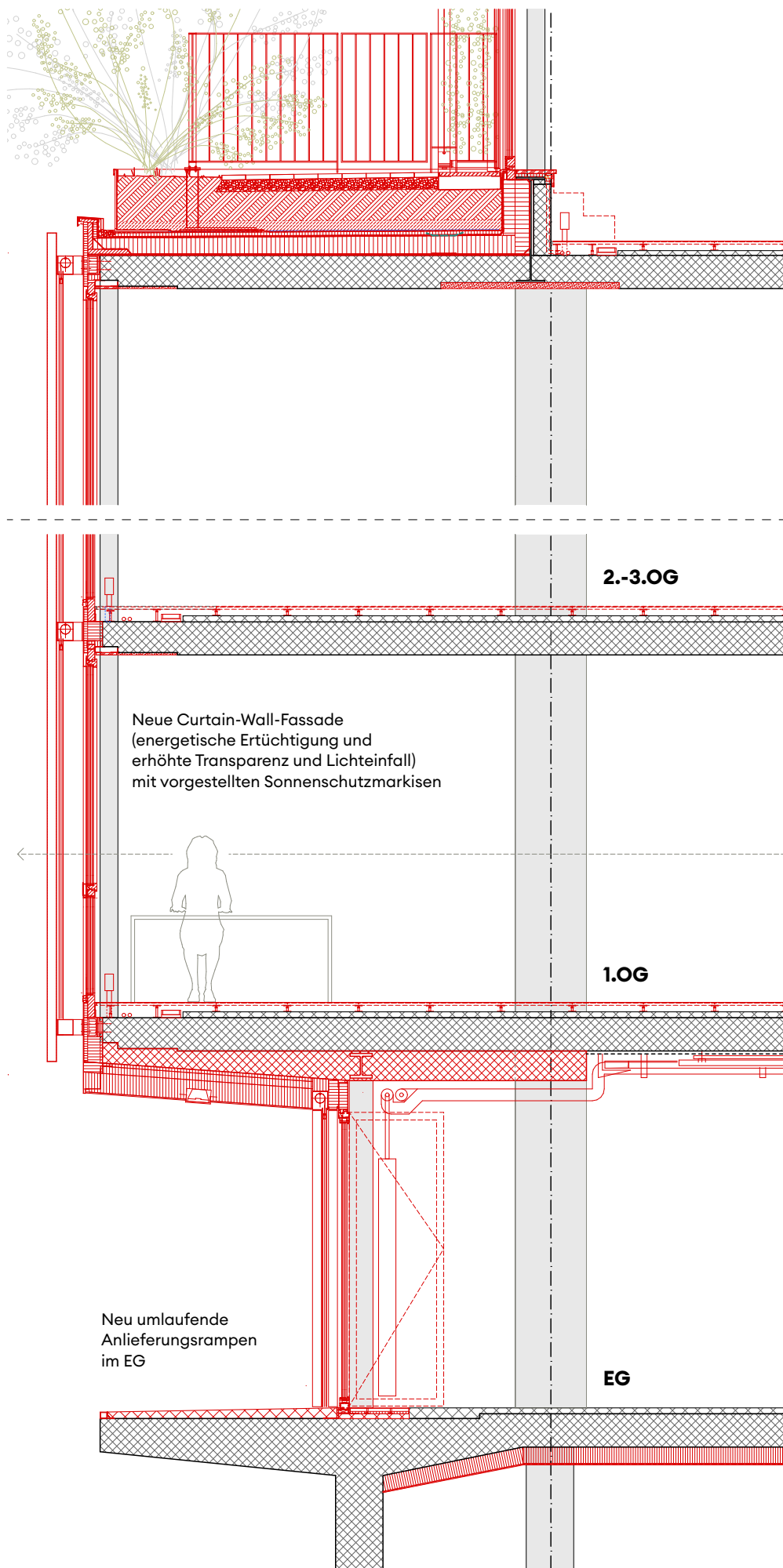
Detailschnitt Erd- Regelgeschoss
