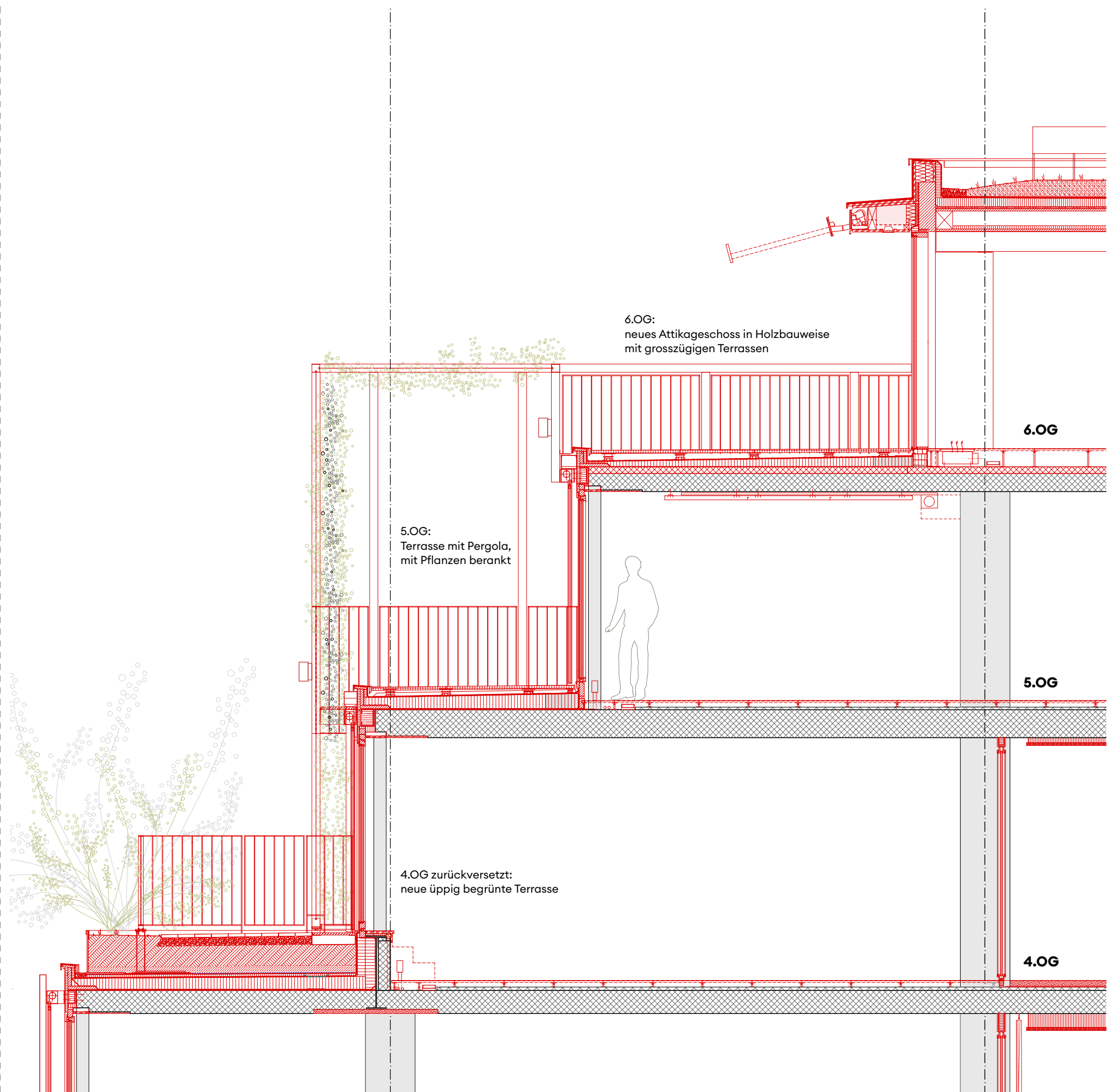
Detailschnitt 4.-5.-6. Obergeschoss
