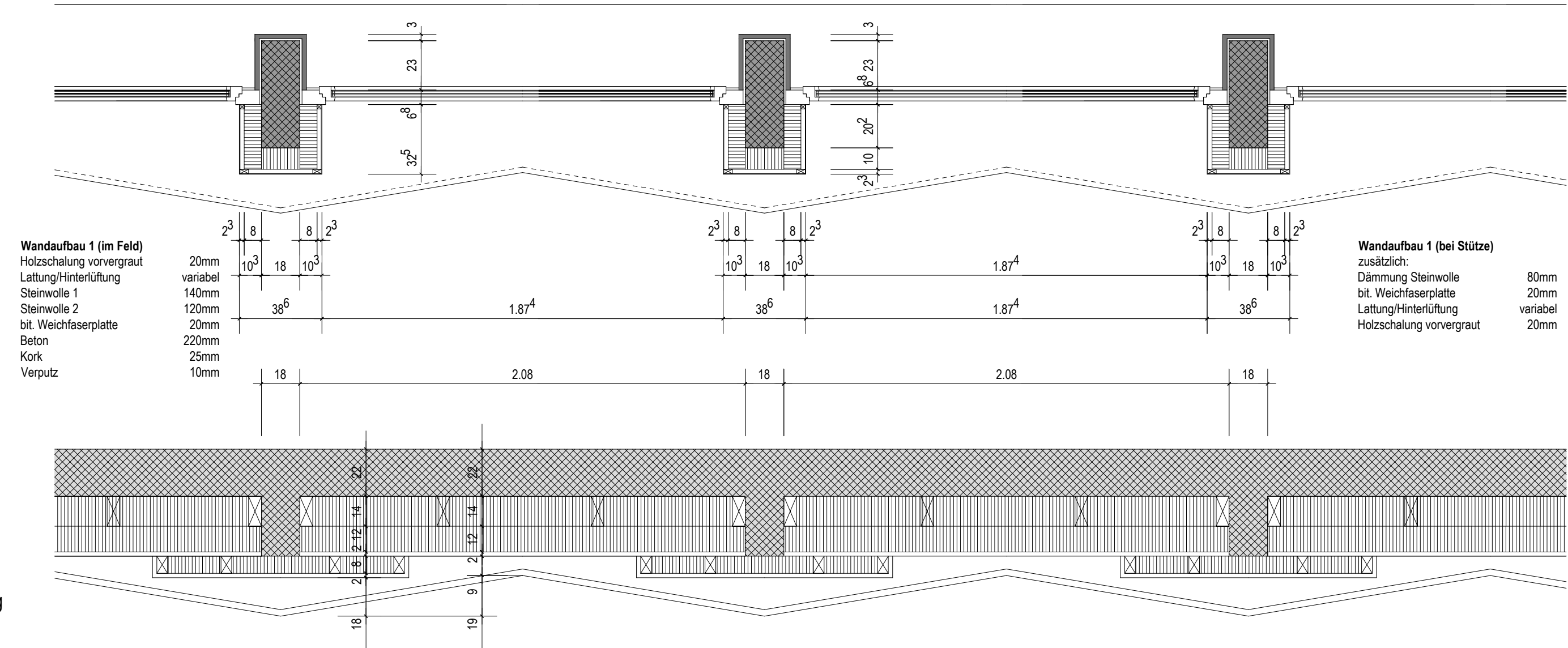
Schnitt Brüstung
