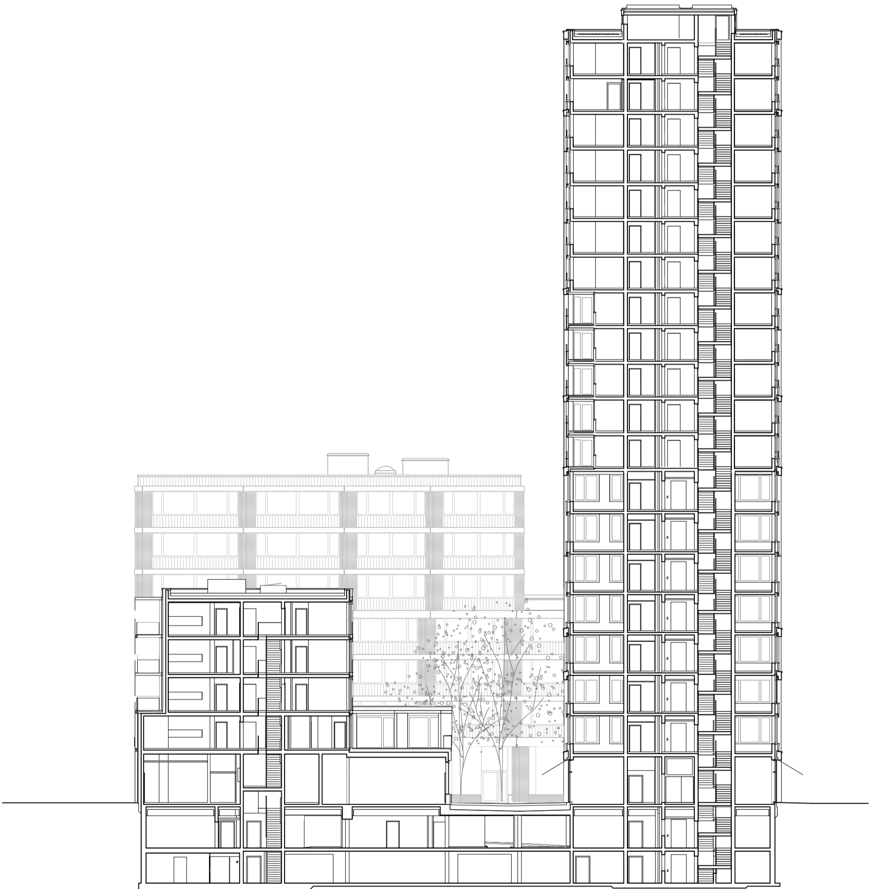
Coupes et élévations sur façades est
