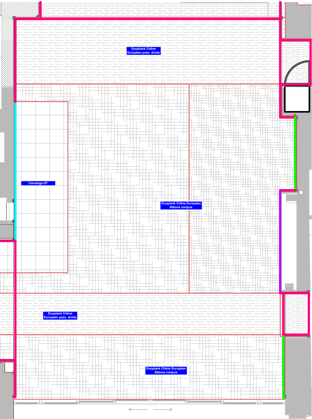
Plan Memorabilia - Revêtements de sols & Murs Echelle : 1-100
