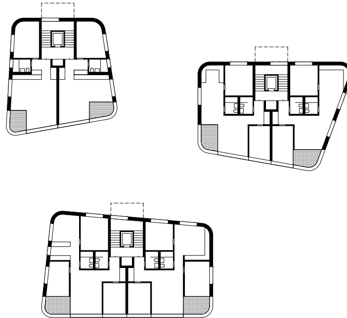
Grundriss DG
