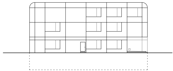
façade est
