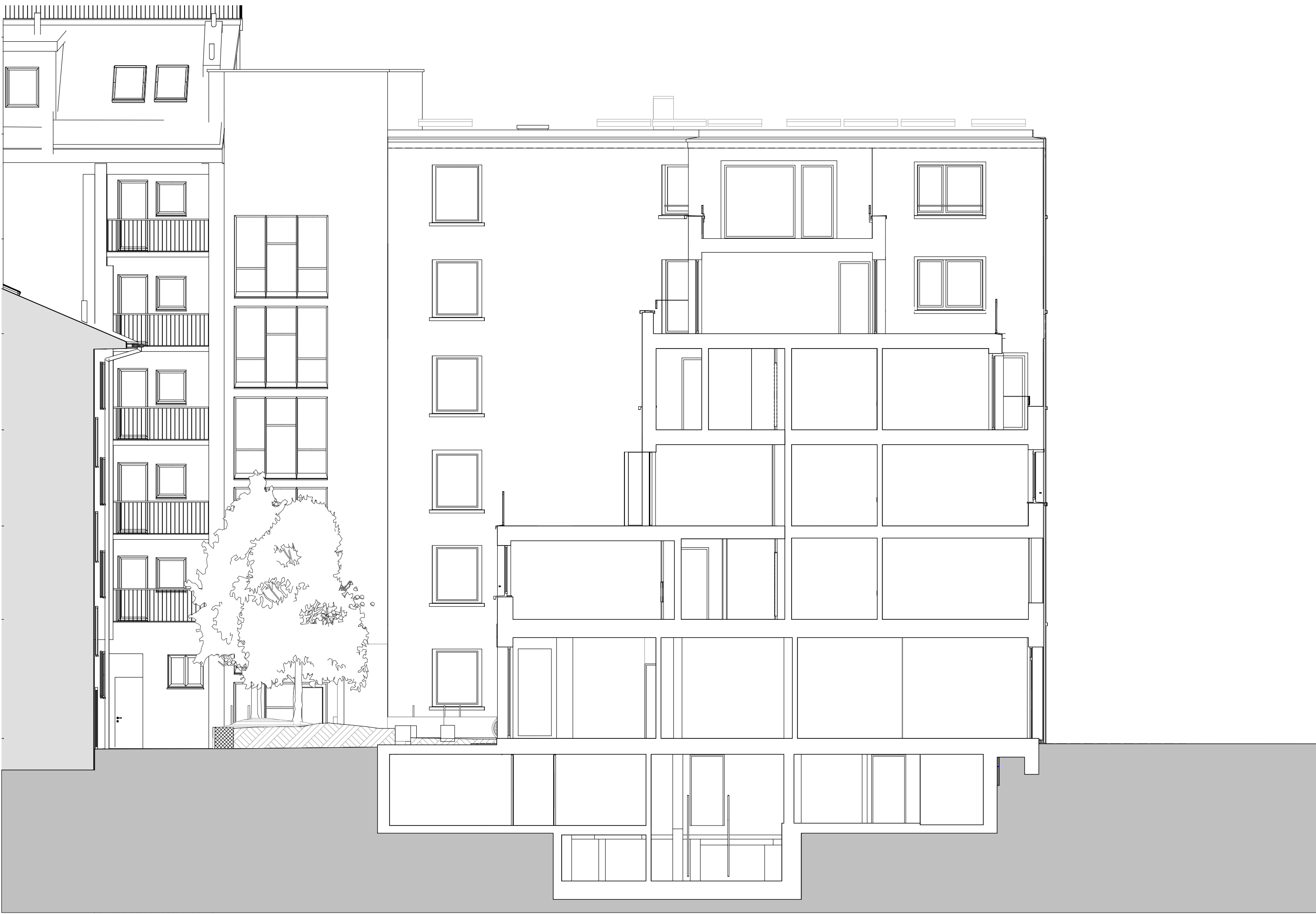
Schnitt
