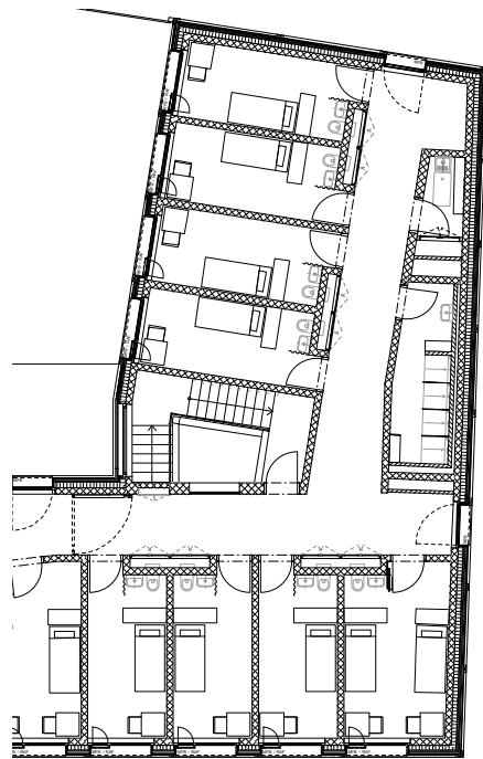
Ausschnitt Wohngruppe Obergeschoss
