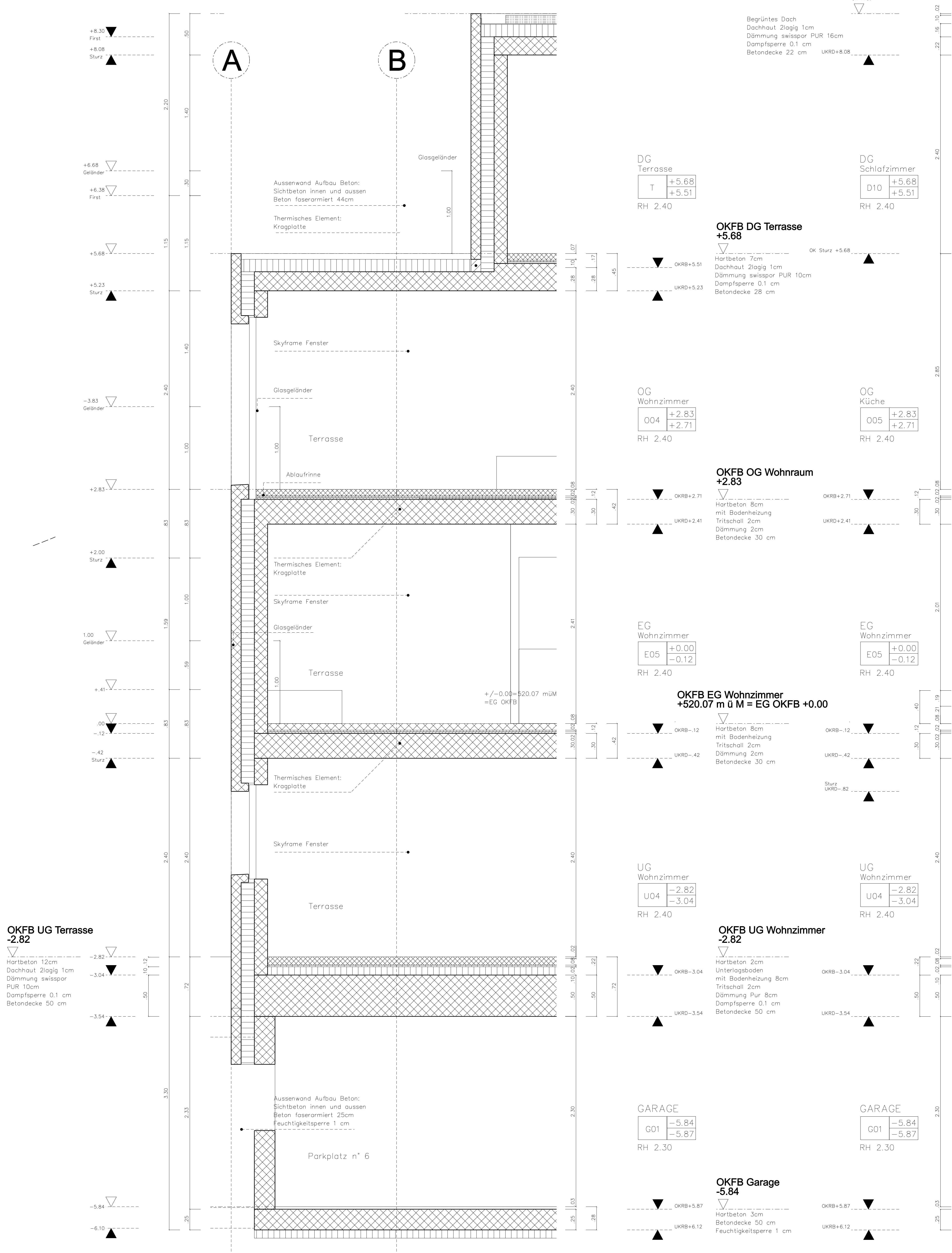
Fassadeschnitt FS2 01
